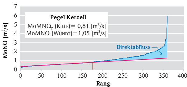
Abb. 7: Abtrennung des Direktabflusses nach KILLE (1970).
