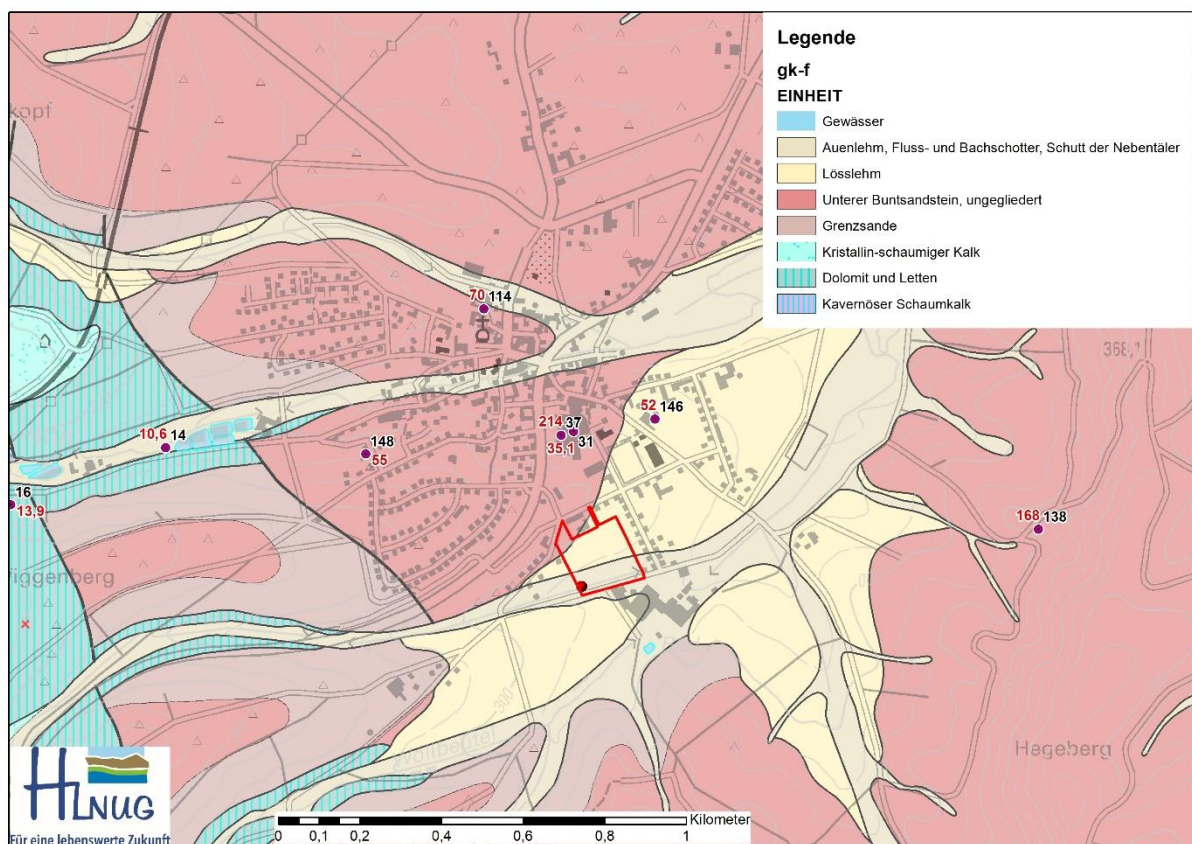
Abb. 3: Ausschnitt aus der digitalen geologischen Karte 1 : 25.000, GK 4619 Mengerlinghausen. Rote Linie: Geltungsbereich, roter Punkt: Erkundungsbohrung. Rote Punkte außerhalb des Baugebiets: Umliegende Bohrungen im Archiv des HLNUG, Schwarze Beschriftung: Archiv-Nr., rote Beschriftung: Teufe
