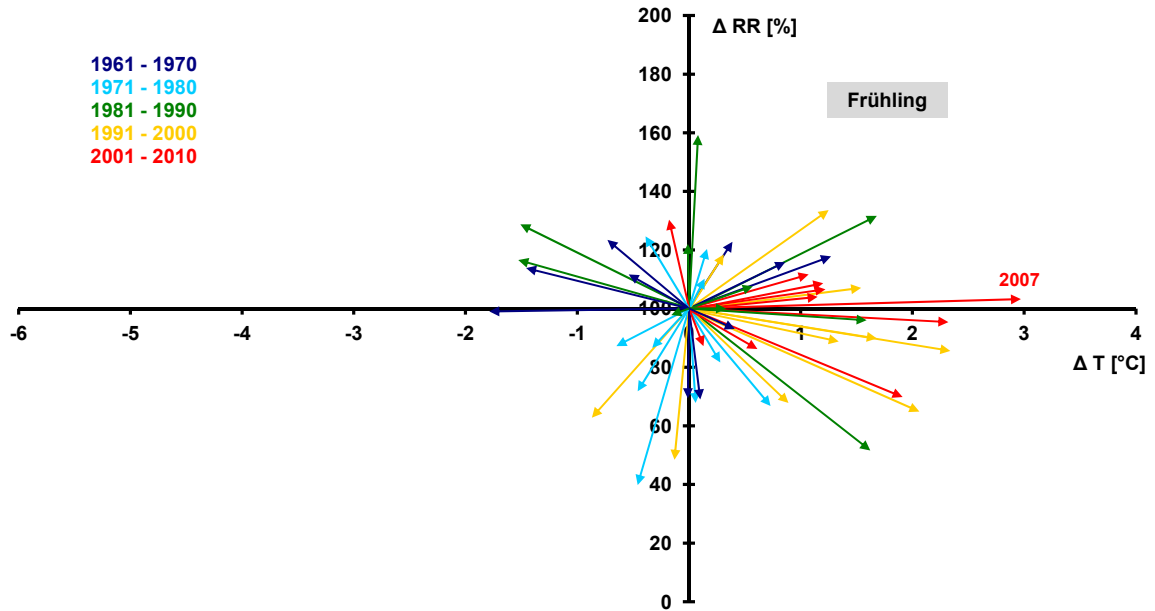
Abb. 11a: Thermopluviogramm Hessen, Abweichung der Jahreswerte gegenüber 1961–1990, Frühling (ΔT: Temperaturdifferenz, ΔRR: Niederschlagsdifferenz) [DWD, 2011]
