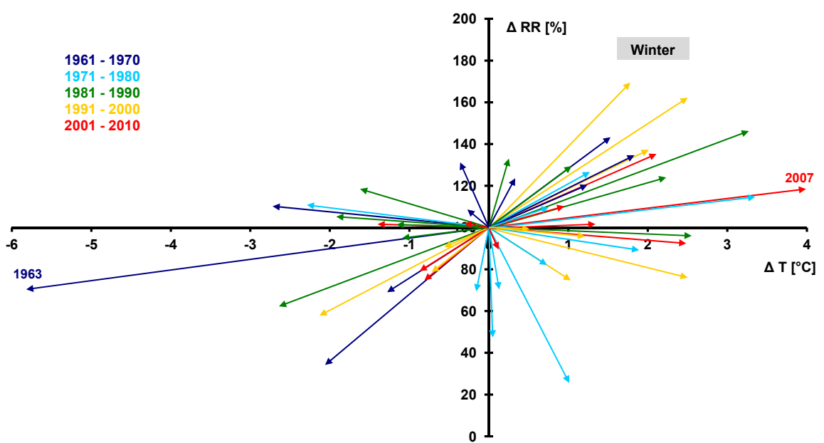
Abb. 11d: Thermopluviogramm Hessen, Abweichung der Jahreswerte gegenüber 1961–1990, Winter ( \Delta T : Temperaturdifferenz, \Delta RR : Niederschlagsdifferenz) [DWD, 2011]
