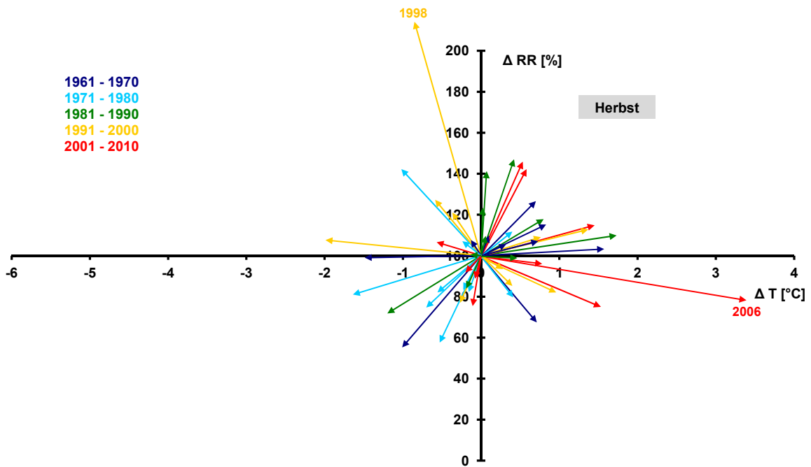
Abb. 11c: Thermopluviogramm Hessen, Abweichung der Jahreswerte gegenüber 1961–1990, Herbst ( \Delta T : Temperaturdifferenz, \Delta RR : Niederschlagsdifferenz) [DWD, 2011]
