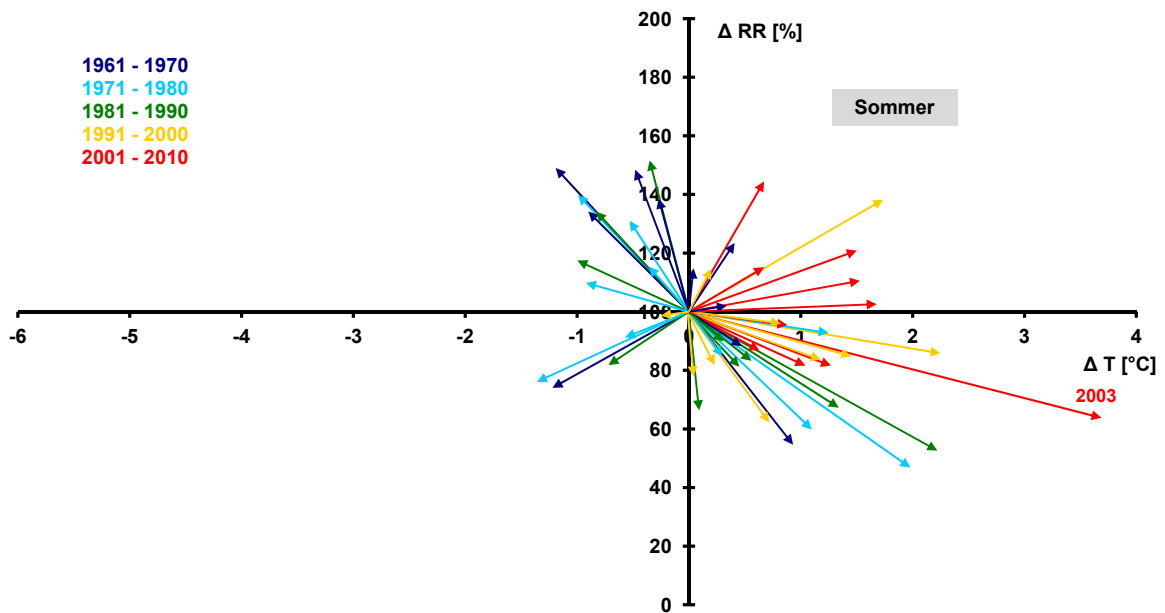
Abb. 11b: Thermopluviogramm Hessen, Abweichung der Jahreswerte gegenüber 1961–1990, Sommer (ΔT: Temperaturdifferenz, ΔRR: Niederschlagsdifferenz) [DWD, 2011]
