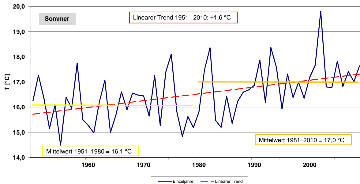
Abb. 4b: Mitteltemperatur (T) (Hessen-Gebietsmittel), 1951–2010, Sommer [DWD, 2011]
