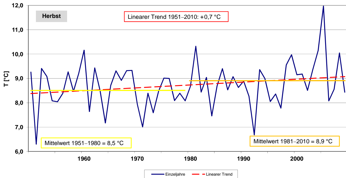
Abb. 4c: Mitteltemperatur (T) (Hessen-Gebietsmittel), 1951–2010, Herbst [DWD, 2011]
