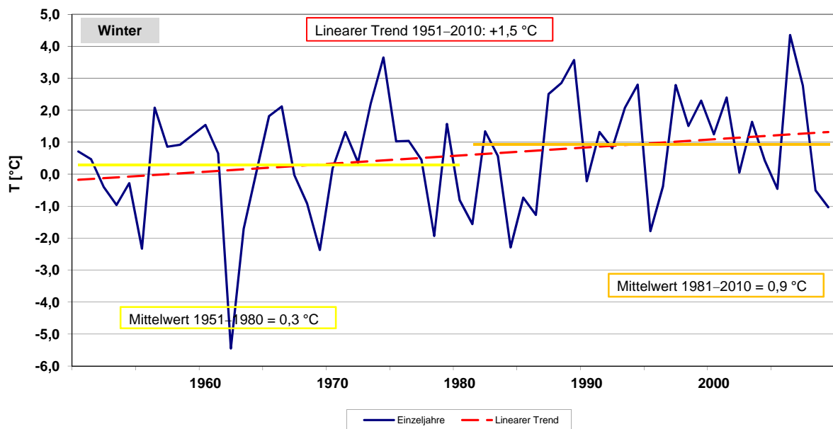
Abb. 4d: Mitteltemperatur (T) (Hessen-Gebietsmittel), 1951–2010, Winter [DWD, 2011]
