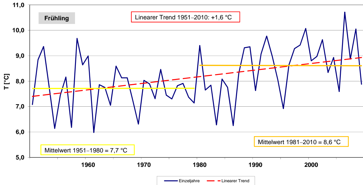
Abb. 4a: Mitteltemperatur (T) (Hessen-Gebietsmittel), 1951–2010, Frühling [DWD, 2011]
