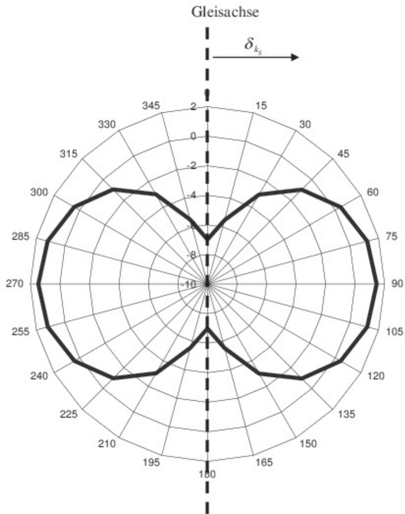
Bild 3: Richtwirkungsmaß D_{I,KS} in dB nach Gleichung (Gl. 8) für \delta_{KS} in Grad
