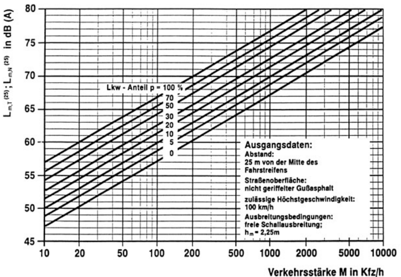
Diagramm I : Mittelungspegel L_{m,T}^{(25)} bzw. L_{m,N}^{(25)} in dB (A)
