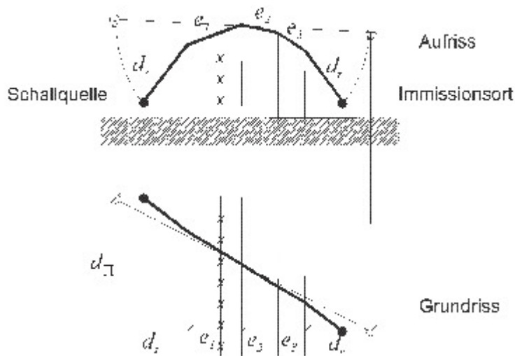
Bild 6: Beispiel für einen Schallweg über mehr als zwei maßgebliche parallele Beugungskanten; zu vernachlässigende Kanten sind durch x markiert Die Auswahl der maßgeblichen Beugungskanten erfolgt nach der sogenannten Gummibandmethode. Kanten, die von einem Gummiband, das von der Punktschallquelle zum Immissionsort gespannt wird, nicht berührt werden, bleiben für die Mehrfachbeugung unberücksichtigt. Bei nicht parallelen Beugungskanten, d. h. wenn mindestens eine Beugungskante nicht parallel zu den übrigen am Gummiband beteiligten Beugungskanten ist, gilt:
