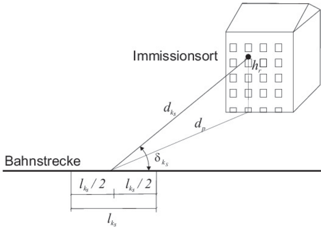
Bild 2: Definition des Winkels \delta_{k_s} an einer Bahnstrecke
