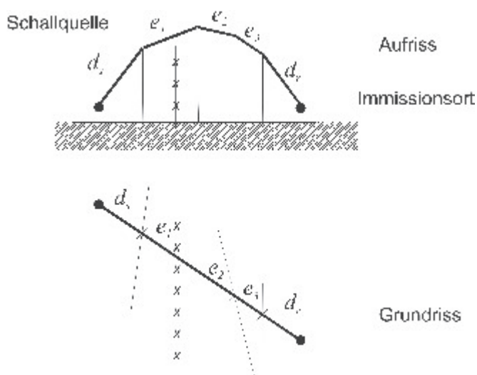
Bild 7: Beispiel für einen Schallweg über mehr als zwei maßgebliche nicht parallele Beugungskanten; zu vernachlässigende Kanten sind durch x markiert Mehrfachbeugung wird nur berücksichtigt, wenn der Weg des gebeugten Schalls, wie in Bild 6 beispielhaft dargestellt, über mehrere Kanten führt.
