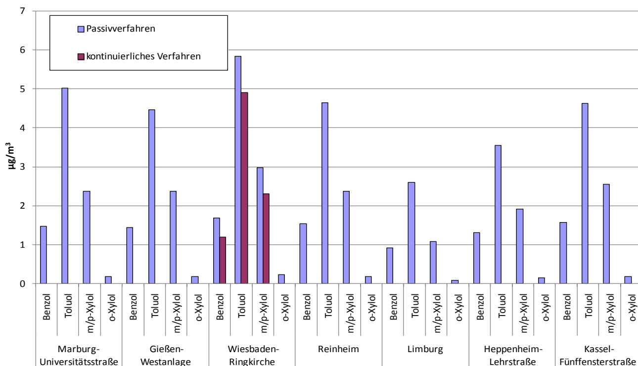
Abbildung 7: Jahresmittelwerte der BTX-Konzentration erhoben nach der Passivsammelverfahren sowie Vergleich mit den Ergebnissen des kontinuierlich registrierenden BTX-Messplatzes
