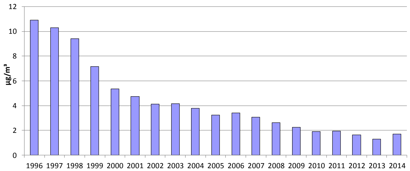
Abbildung 8 : Zeitliche Entwicklung der Benzol-Jahresmittelwerte, Station Wiesbaden-Ringkirche (Erhebung mit kontinuierlich messendem BTX-Analysator)
