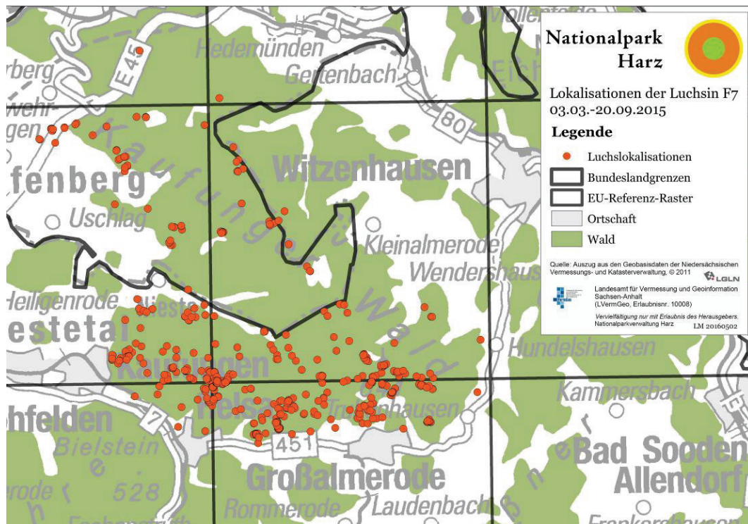
Abb. 6: Streifgebiet der Luchs F7, ermittelt per GPS-Telemetrie durch das Luchsprojekt Harz. Karte freundlicherweise zur Verfügung gestellt vom LUCHSPROJEKT HARZ.
