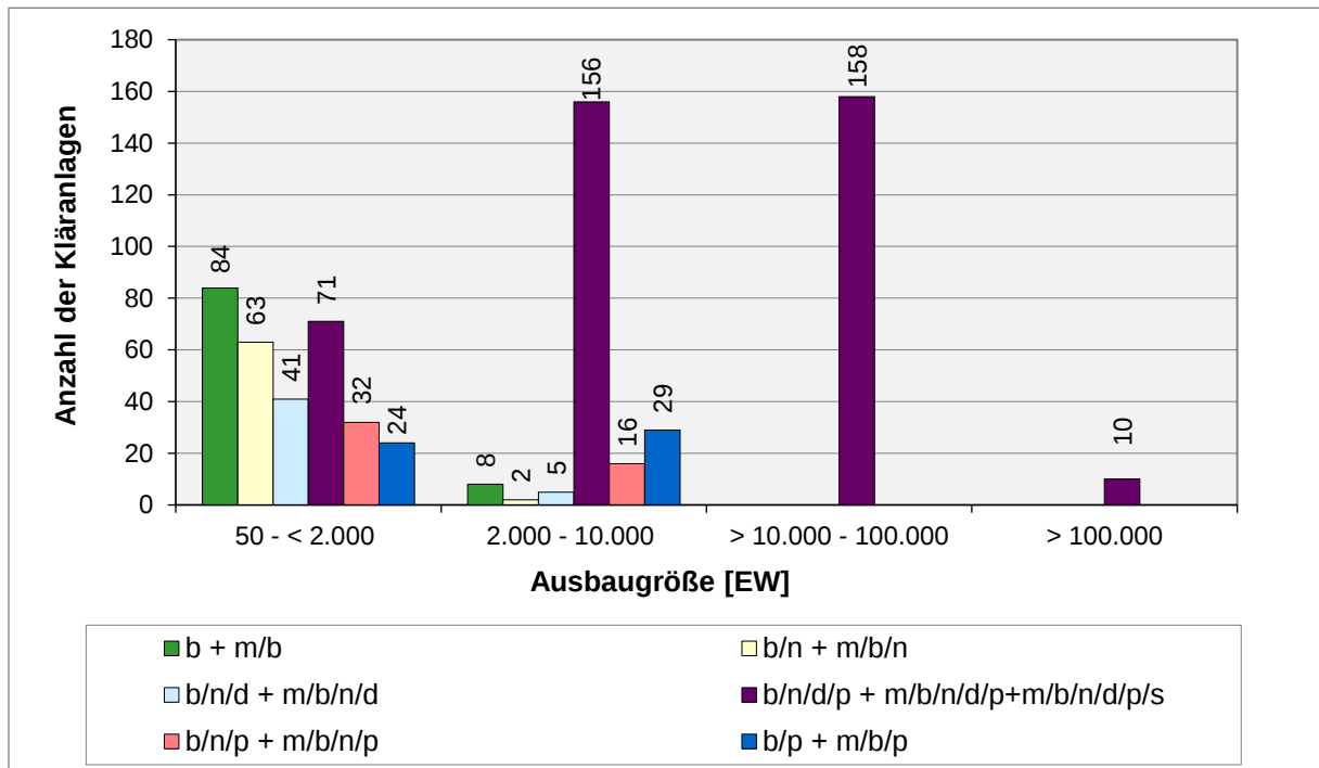
Abb. 8: Aktueller Verfahrensstand (Reinigungsart/-stufen) der hessischen Kläranlagen gegliedert nach Ausbaugrößen (Stand: 31.12.2024)
