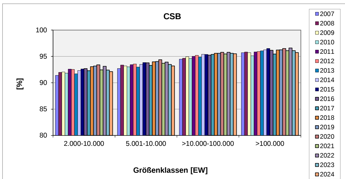
Abb. 15: Abbau-/Eliminationsraten hessischer Kläranlagen in den Jahren von 2007 bis 2024 für den Parameter CSB (Grundlage: Eigenkontrolldaten)
