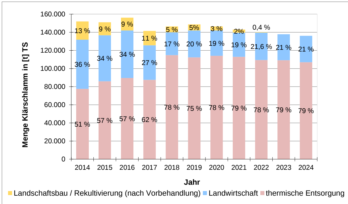
Abb. 25: Prozentuale Verteilung der entsorgten Klärschlamm-mengen nach Entsorgungswegen in den Jahren 2014 bis 2024 – bezogen auf alle kommunalen Kläranlagen mit einer Ausbaugröße ab 50 EW
