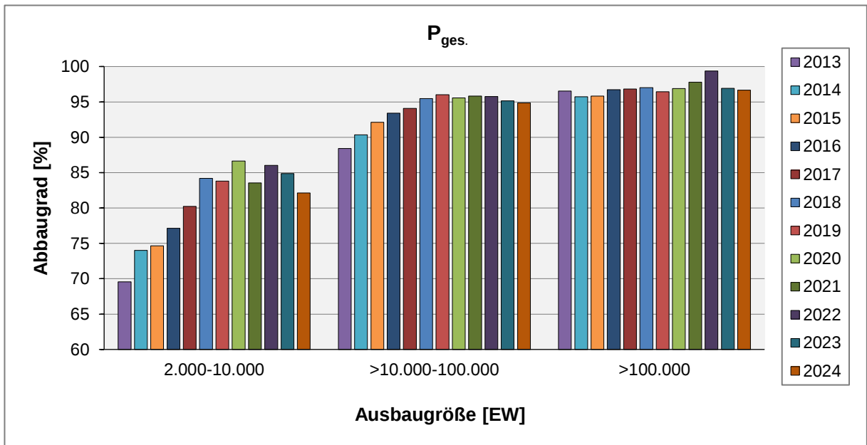
Abb. 23: Abbaugrad (Reinigungsleistung) hessischer Kläranlagen hinsichtlich des Parameters P_{\text{ges.}} in den Jahren 2013 bis 2024 (Ergebnisse der staatlichen Überwachung)
