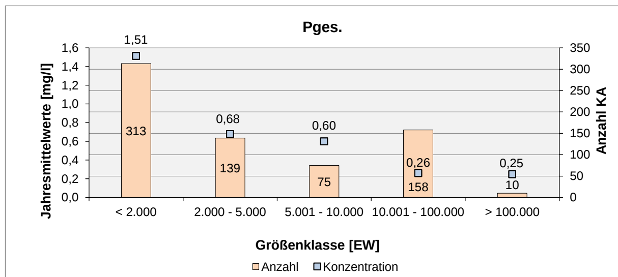
Abb. 21: Ablaufkonzentration im Jahresmittel für den Parameter P_{\text{ges.}} im Jahr 2024
