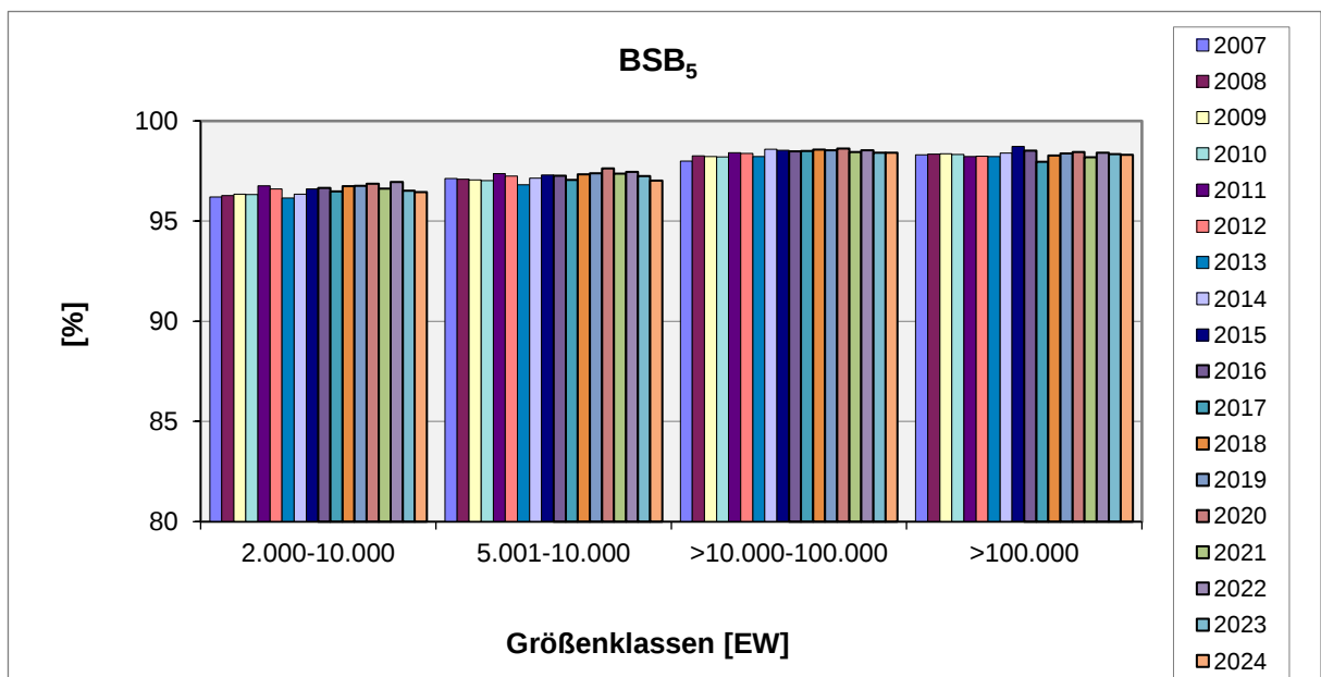
Abb. 14: Abbau-/Eliminationsraten hessischer Kläranlagen in den Jahren von 2007 bis 2024 für den Parameter BSB 5 (Grundlage: Eigenkontrolldaten)
