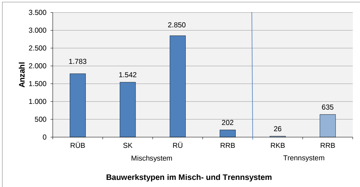
Abb. 4: Anzahl der Regenbecken und Entlastungsanlagen nach Bauwerksart
