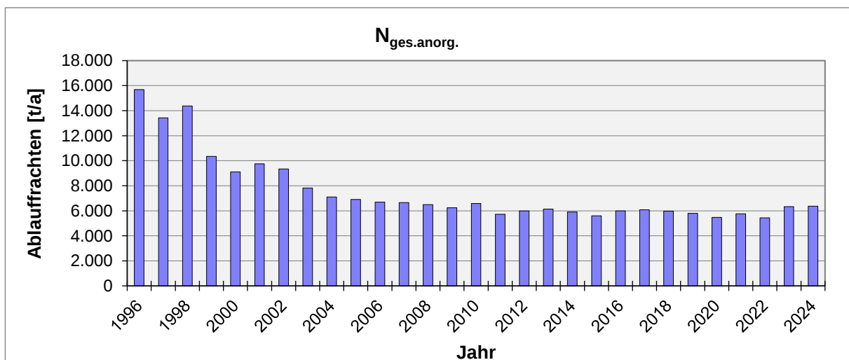
Abb. 11: Jahresablauffrachten von 1996 bis 2024 in [t/Jahr], Parameter N ges.anorg.
