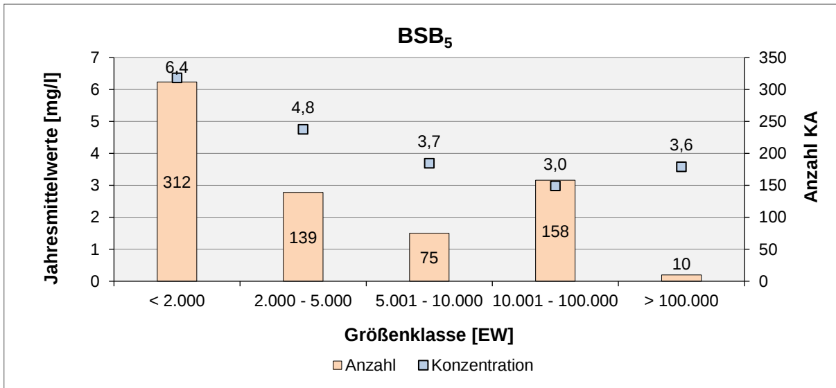
Abb. 18: Ablaufkonzentration im Jahresmittel für den Parameter BSB 5 im Jahr 2024
