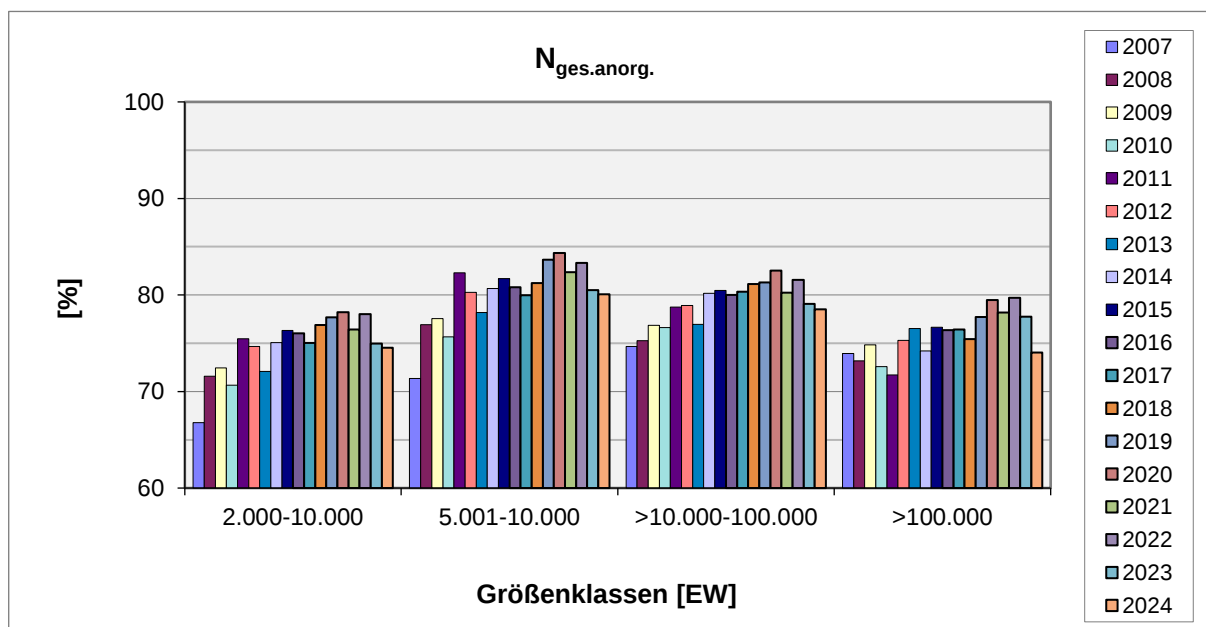
Abb. 16: Abbau-/Eliminationsraten hessischer Kläranlagen in den Jahren von 2007 bis 2024 für den Parameter N_{\text{ges.anorg.}} (Grundlage: Eigenkontrolldaten)
