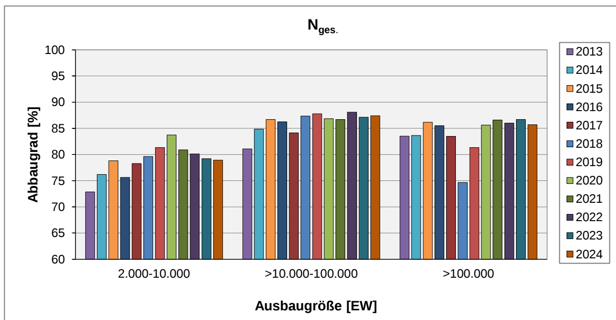
Abb. 22: Abbaugrad (Reinigungsleistung) hessischer Kläranlagen hinsichtlich des Parameters Gesamtstickstoff N_{ges.}^* in den Jahren 2013 bis 2024 (Ergebnisse der staatlichen Überwachung) ^* N_{ges.} = (N_{org.} + NH_4-N + NO_3-N + NO_2-N)
