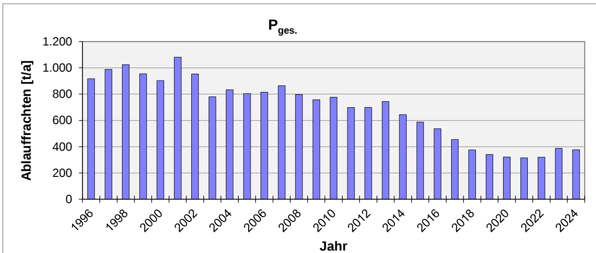
Abb. 12: Jahresablauffrachten von 1996 bis 2024 in [t/Jahr], Parameter P_{ges.}
