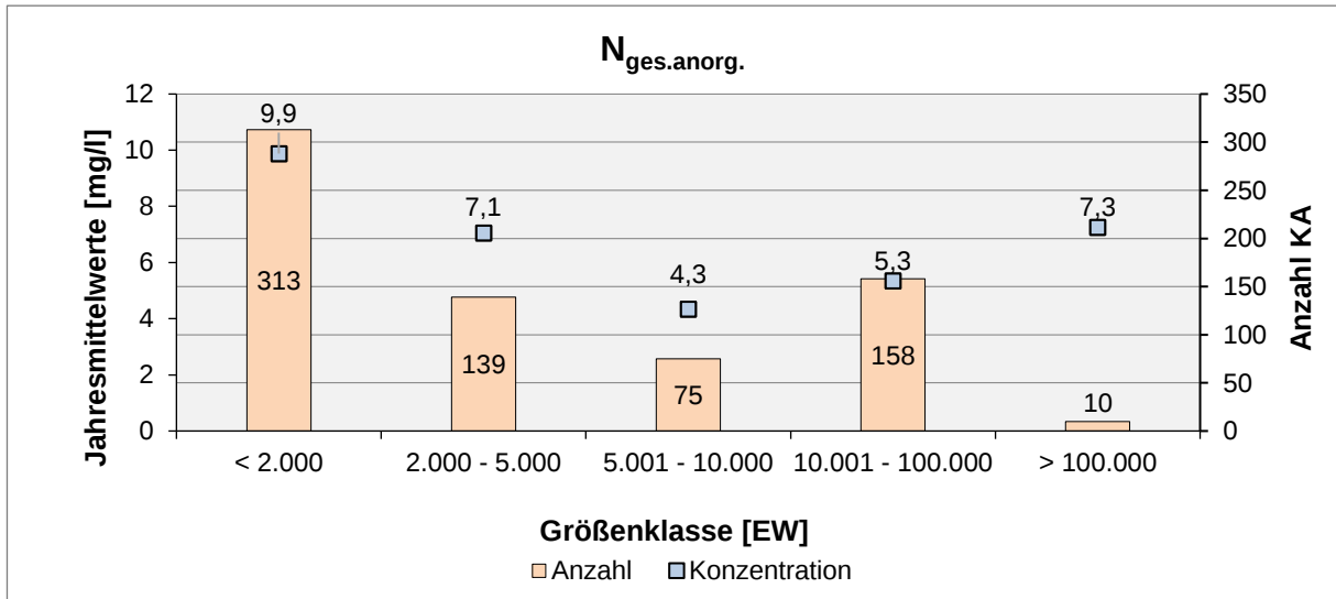
Abb. 20: Ablaufkonzentration im Jahresmittel für den Parameter N_{\text{ges.anorg.}} im Jahr 2024
