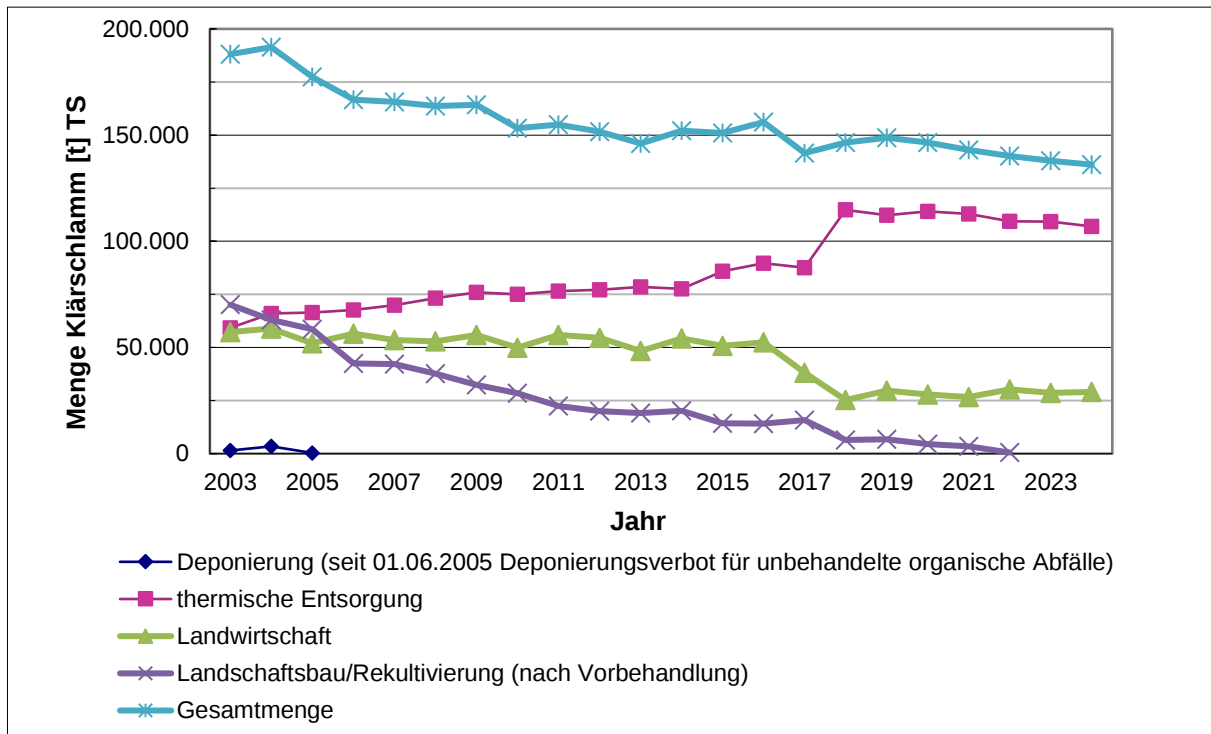
Abb. 24: Entsorgungswege hessischer Klärschlämme in den Jahren 2003 bis 2024
