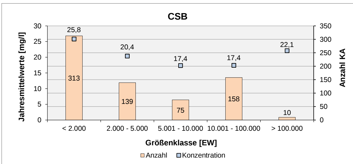
Abb. 19: Ablaufkonzentration im Jahresmittel für den Parameter CSB im Jahr 2024
