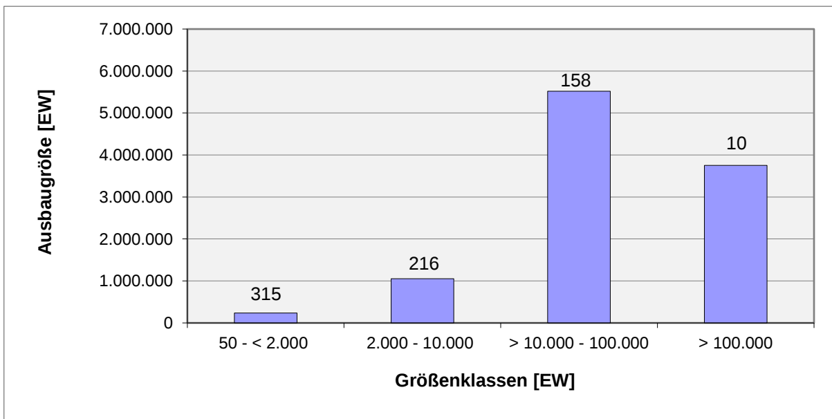
Abb. 6: Anzahl der kommunalen Kläranlagen in Hessen pro Größenklasse (Stand 31.12.2024), bezogen auf deren Ausbaugrößen (EW)
