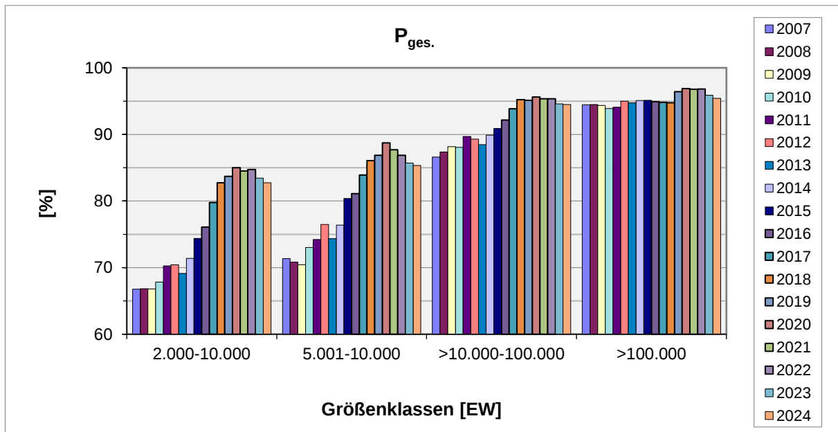
Abb. 17: Abbau-/Eliminationsraten hessischer Kläranlagen in den Jahre von 2007 bis 2024 für den Parameter P_{\text{ges.}} (Grundlage: Eigenkontrolldaten)
