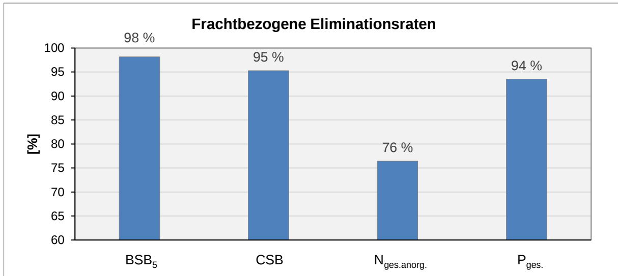
Abb. 13: Frachtbezogene Eliminationsraten der kommunalen Kläranlagen ab 2.000 EW im Jahr 2024 (Grundlage: Eigenkontrolldaten)
