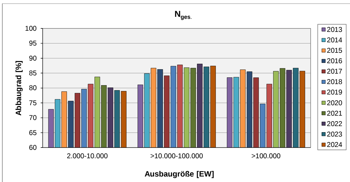
Abb. 22: Abbaugrad (Reinigungsleistung) hessischer Kläranlagen hinsichtlich des Parameters Gesamtstickstoff N_{\text{ges.}} * in den Jahren 2013 bis 2024 (Ergebnisse der staatlichen Überwachung) * N_{\text{ges.}} = (N_{\text{org.}} + \text{NH}_4\text{-N} + \text{NO}_3\text{-N} + \text{NO}_2\text{-N})
