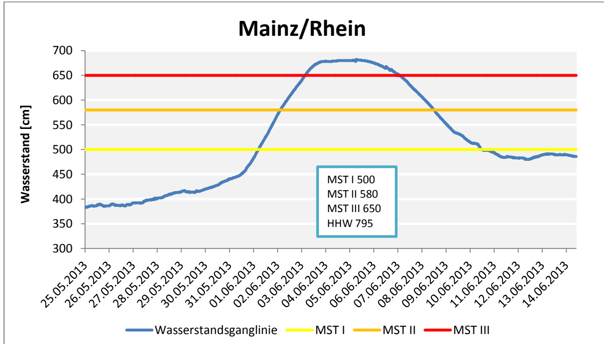
Abb. 33: Wasserstände am Pegel Mainz/Rhein.
