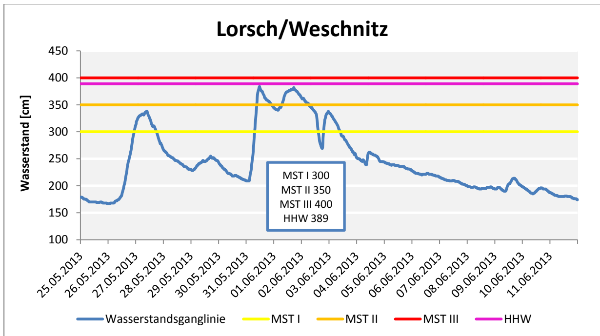
Abb. 11: Wasserstände am Pegel Lorsch/Weschnitz.
