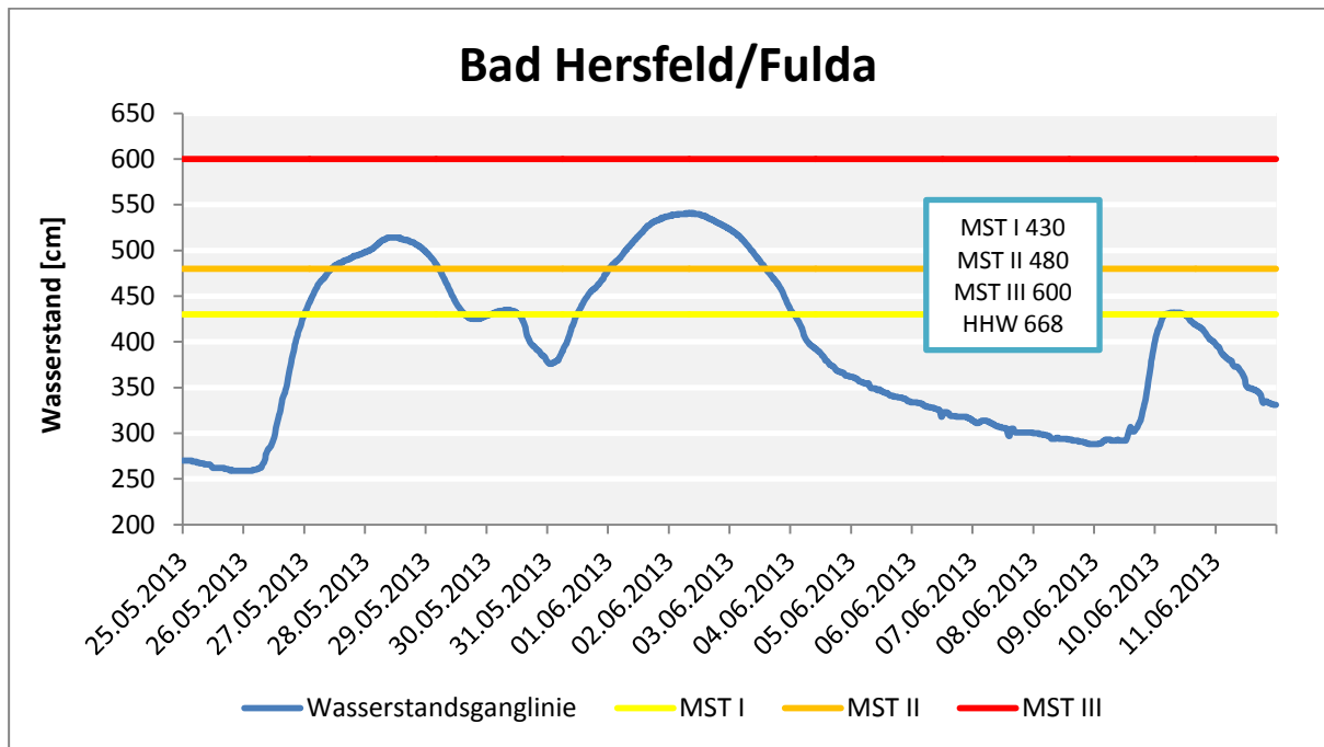
Abb. 27: Wasserstände am Pegel Bad Hersfeld/Fulda.
