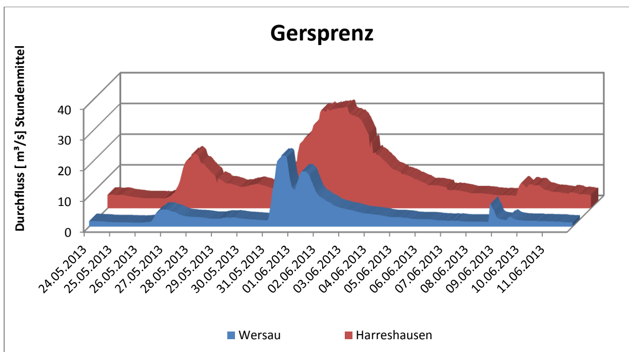
Abb. 12: Durchflüsse an der Gersprenz.
