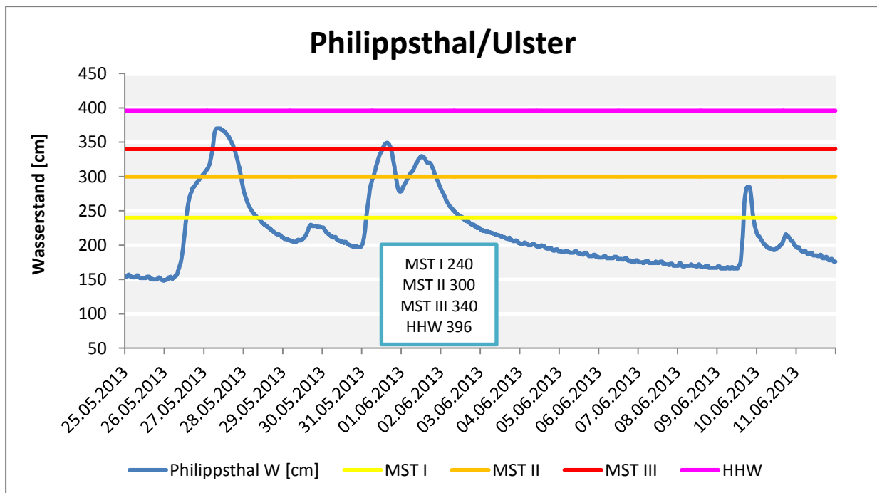
Abb. 23: Wasserstände am Pegel Philippsthal/Ulster.
