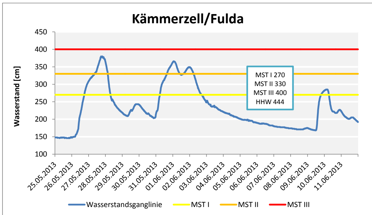
Abb. 26: Wasserstände am Pegel Kämmerzell/Fulda.
