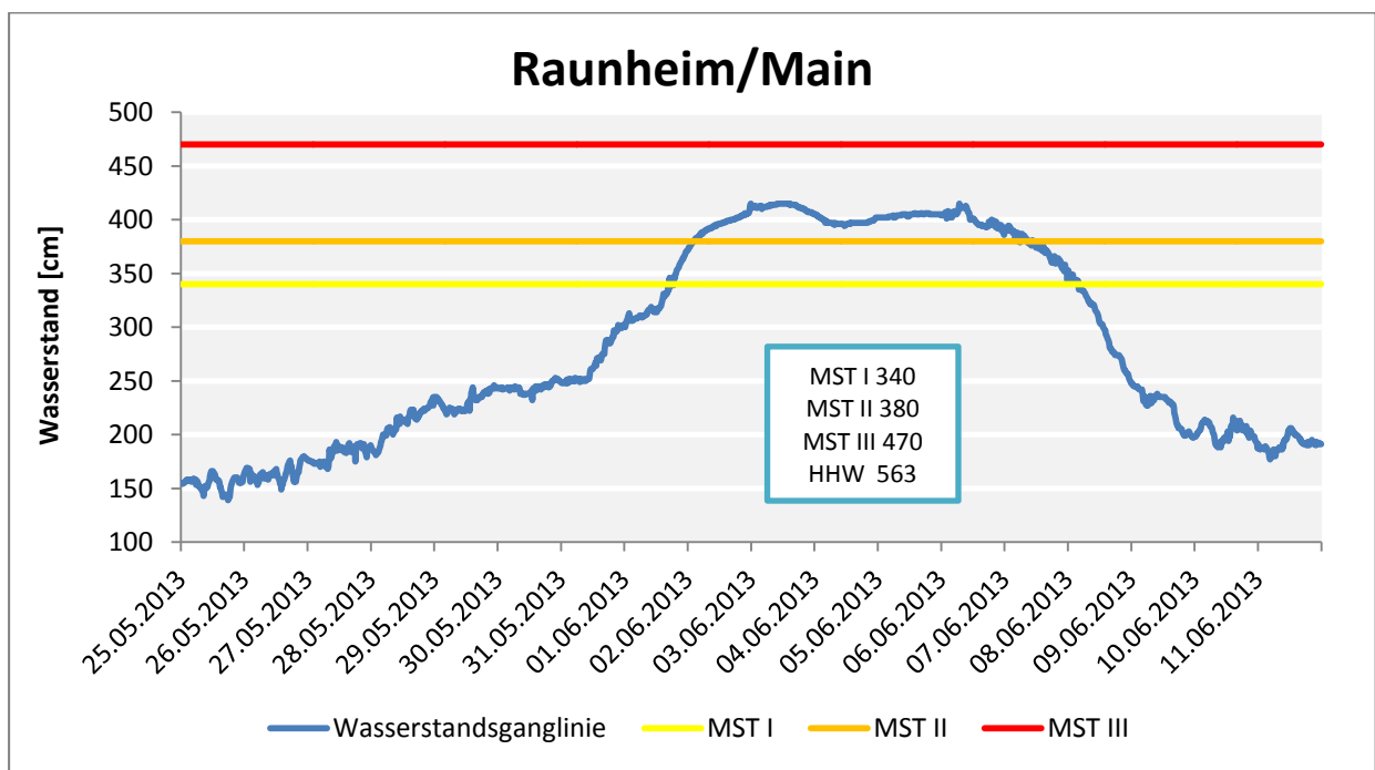
Abb. 39: Wasserstände am Pegel Raunheim/Main.
