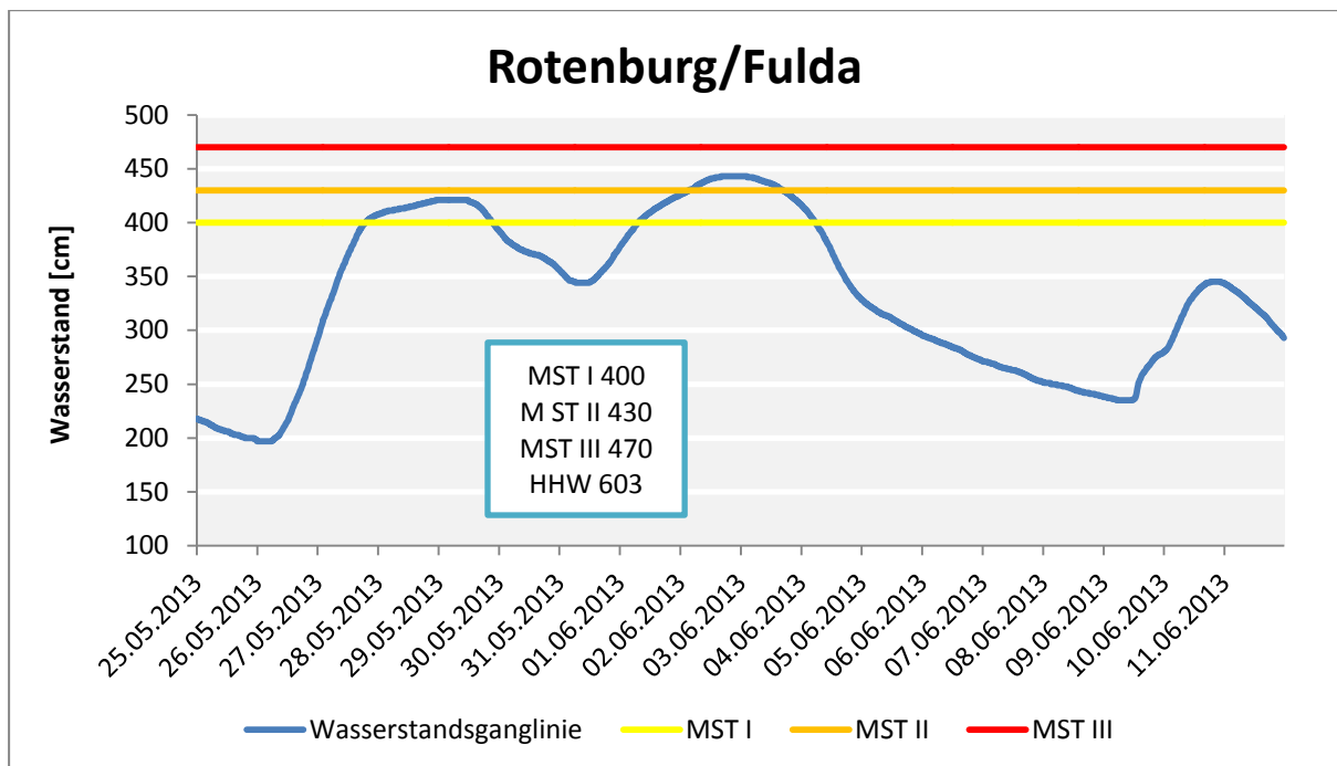
Abb. 28: Wasserstände am Pegel Rotenburg/Fulda.
