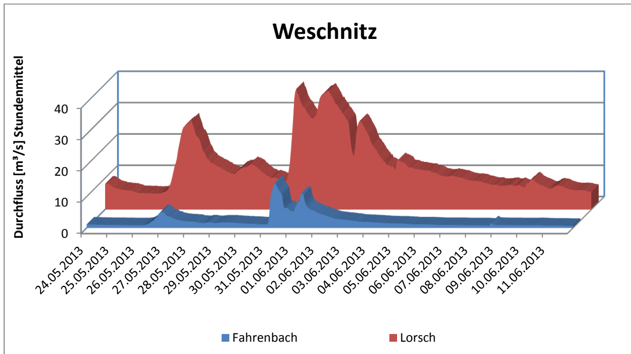
Abb. 10: Durchflüsse an der Weschnitz.
