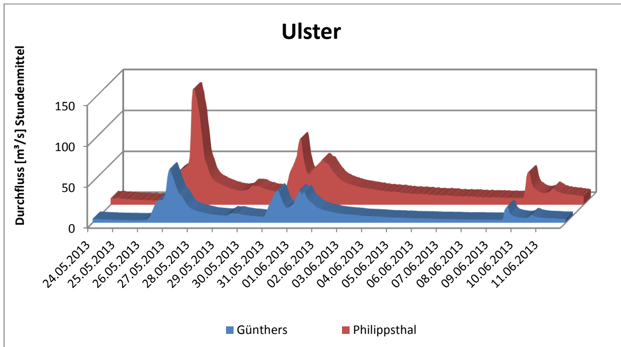
Abb. 22: Durchflüsse an der Ulster.
