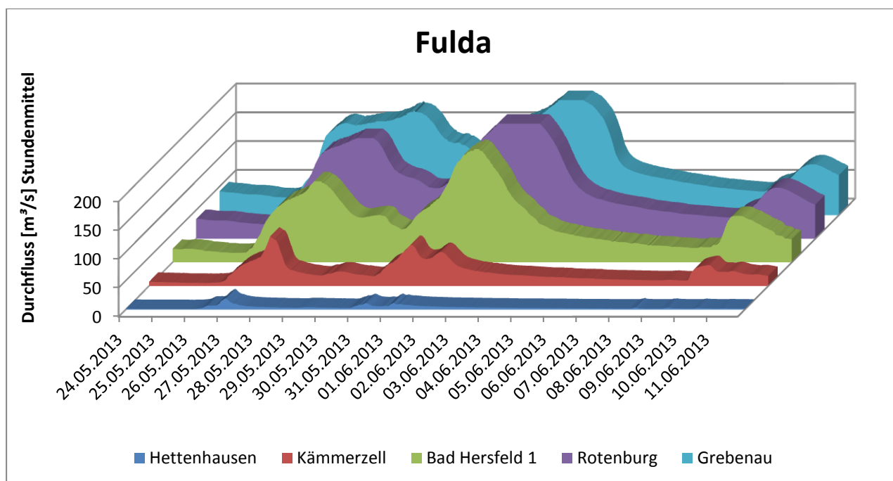
Abb. 24: Durchflüsse an der Fulda.
