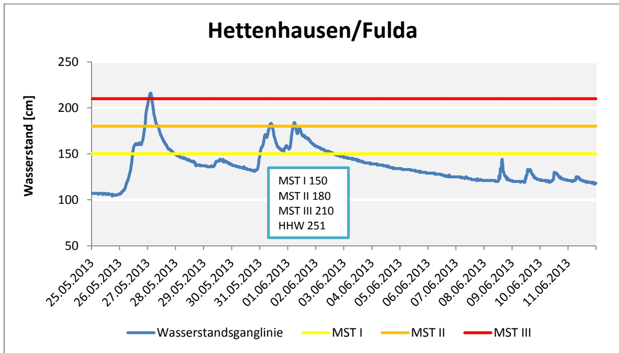
Abb. 25: Wasserstände am Pegel Hettenhausen/Fulda.
