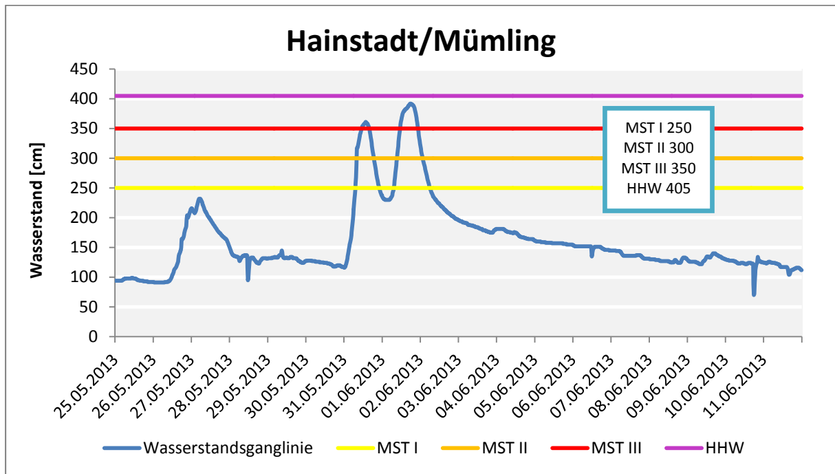
Abb. 9: Wasserstände am Pegel Hainstadt/Mümling.
