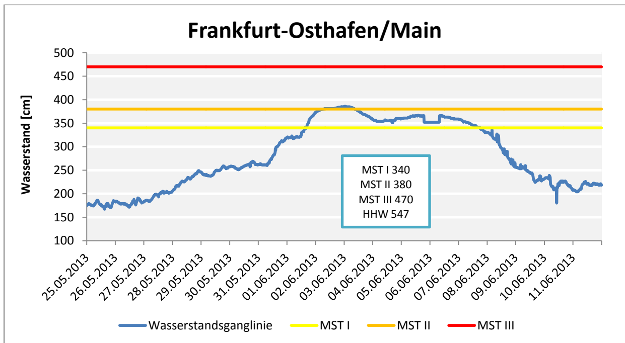
Abb. 38: Wasserstände am Pegel Frankfurt-Osthafen/Main.
