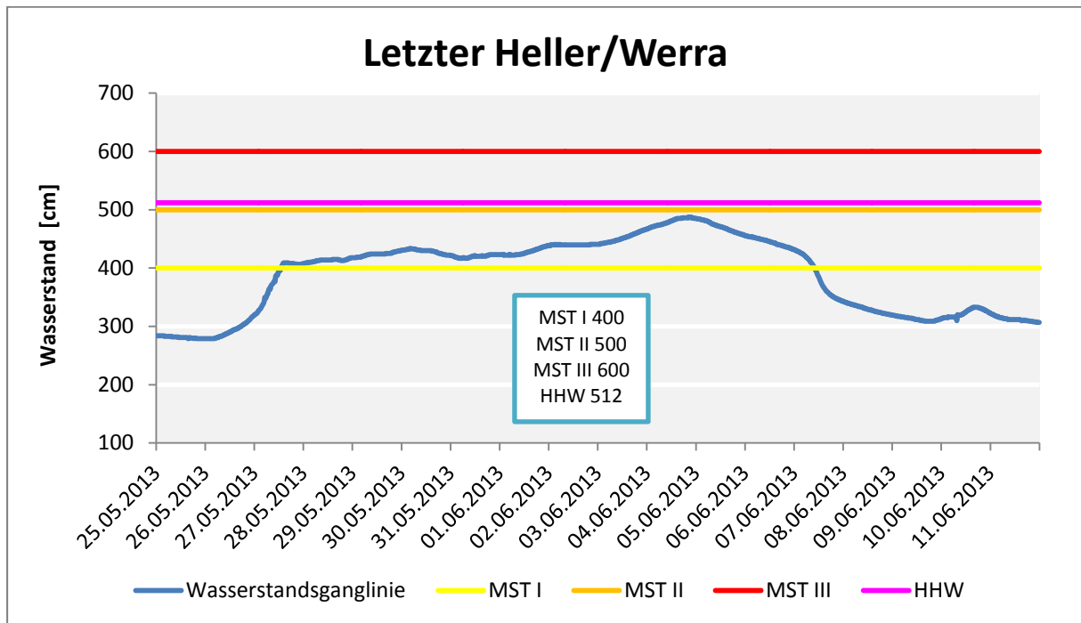
Abb. 21: Wasserstände am Pegel Letzter Heller/Werra.
