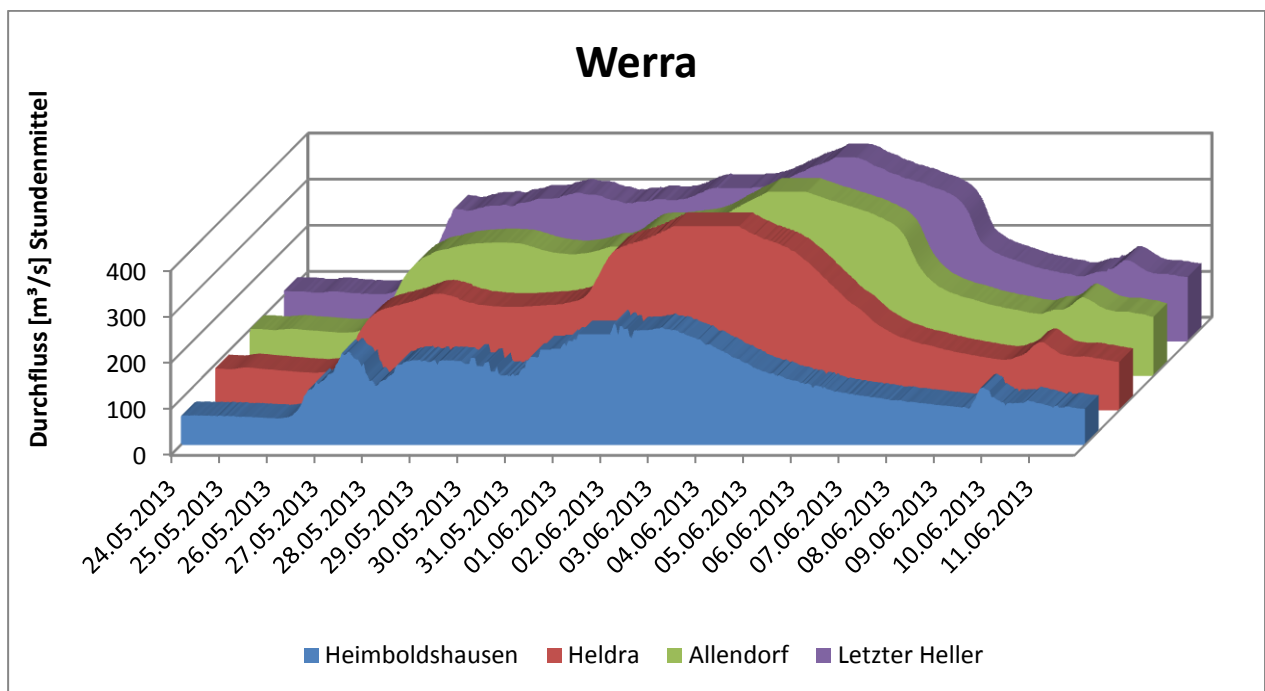
Abb. 14: Durchflüsse an der Werra.
