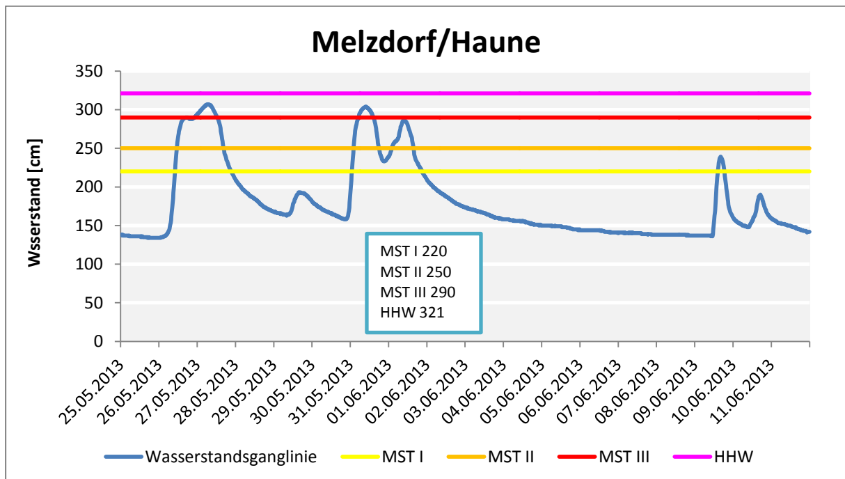
Abb. 30: Wasserstände am Pegel Melzdorf/Haune.
