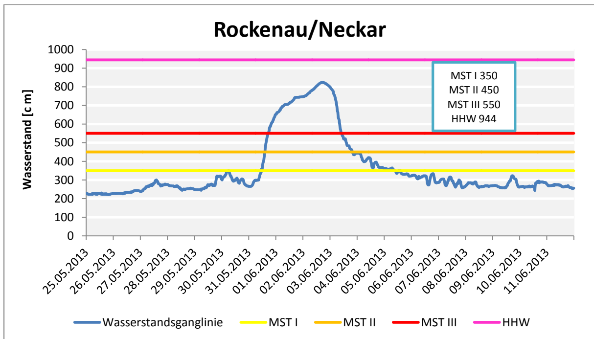
Abb. 42: Wasserstände am Pegel Rockenau/Neckar.
