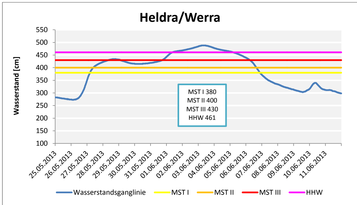
Abb. 17: Wasserstände am Pegel Heldra/Werra.
