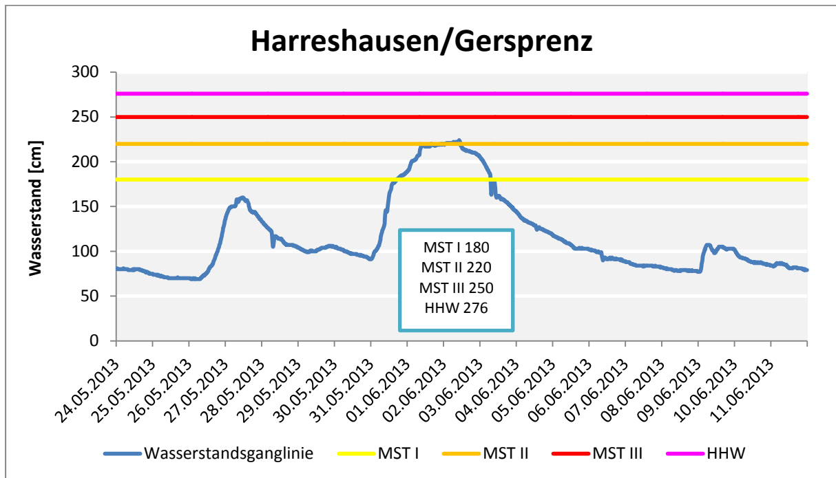
Abb. 13: Wasserstände am Pegel Harreshausen/Gersprenz.
