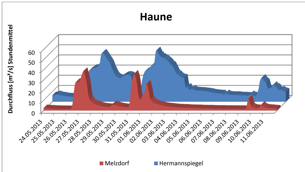
Abb. 29: Durchflüsse an der Haune.
