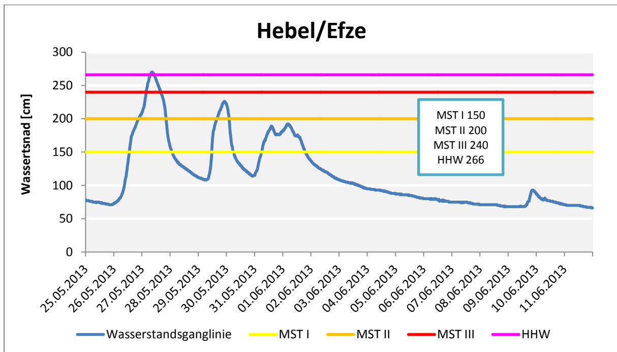
Abb. 31: Wasserstände am Pegel Hebel/Efze.
