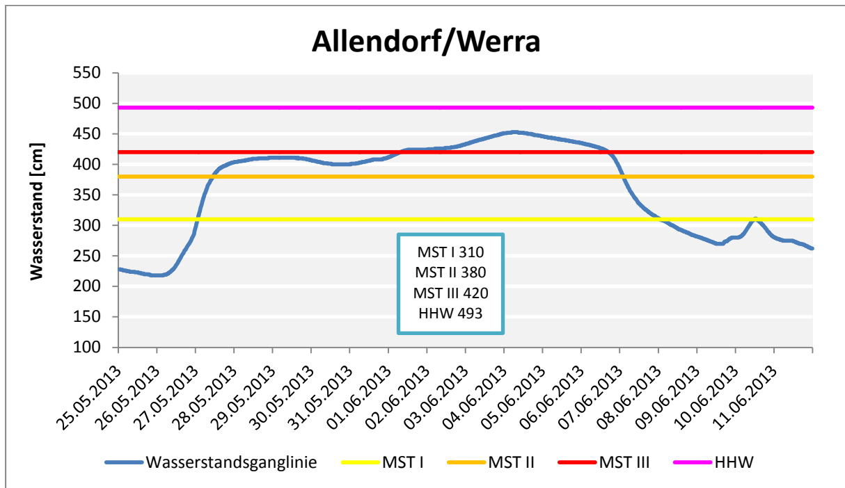
Abb. 19: Wasserstände am Pegel Allendorf/Werra.
