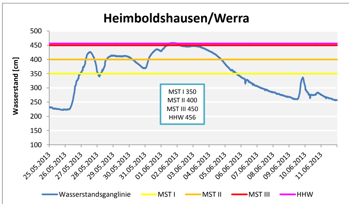
Abb. 16: Wasserstände am Pegel Heimboldshausen/Werra.
