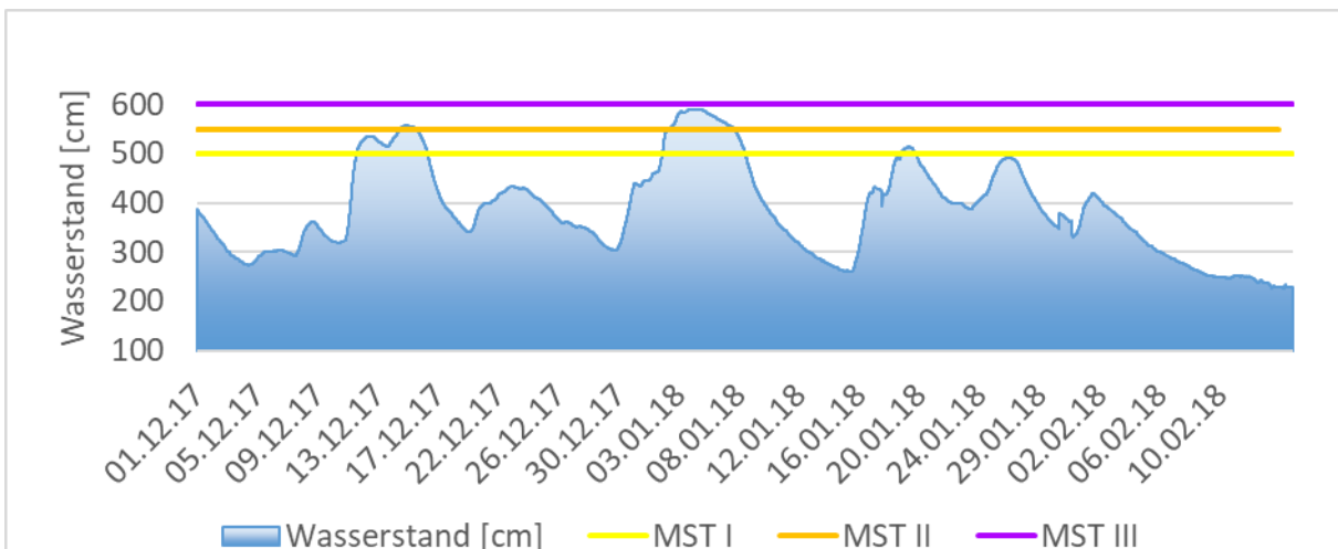
Abbildung 15: Wasserstand am Pegel Leun/ Lahn. Meldestufe 1 = 500 cm (gelbe Linie), Meldestufe 2 = 550 cm (orangefarbene Linie), Meldestufe 3 = 600 cm (lila Linie)
