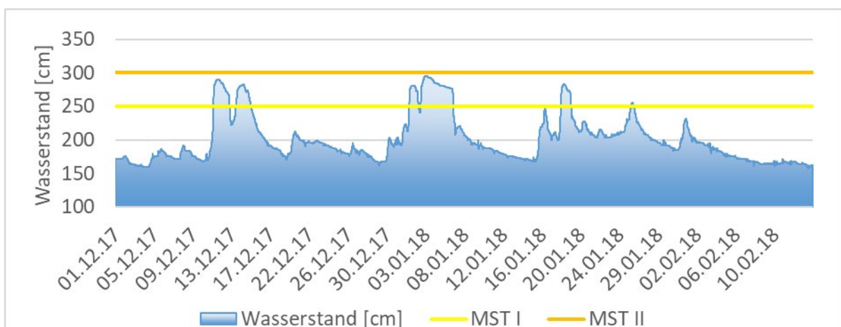
Abbildung 18: Wasserstand am Pegel Bartenhausen / Wohra. Meldestufe 1 = 250 cm (gelbe Linie), Meldestufe 2 = 300 cm (orangefarbene Linie), Meldestufe 3 = 350 cm (nicht in Grafik zu sehen)
