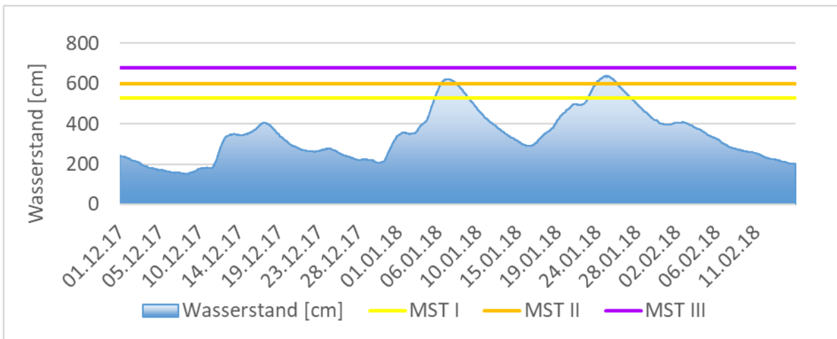
Abbildung 30: Wasserstand am Pegel Worms / Rhein. Meldestufe 1 = 530 cm (gelbe Linie), Meldestufe 2 = 600 cm (orangefarbene Linie), Meldestufe 3 = 680 cm (lila Linie)
