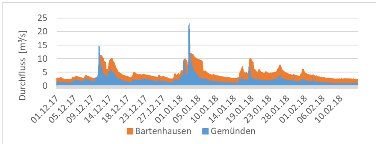
Abbildung 16: Durchflüsse der Wohra
