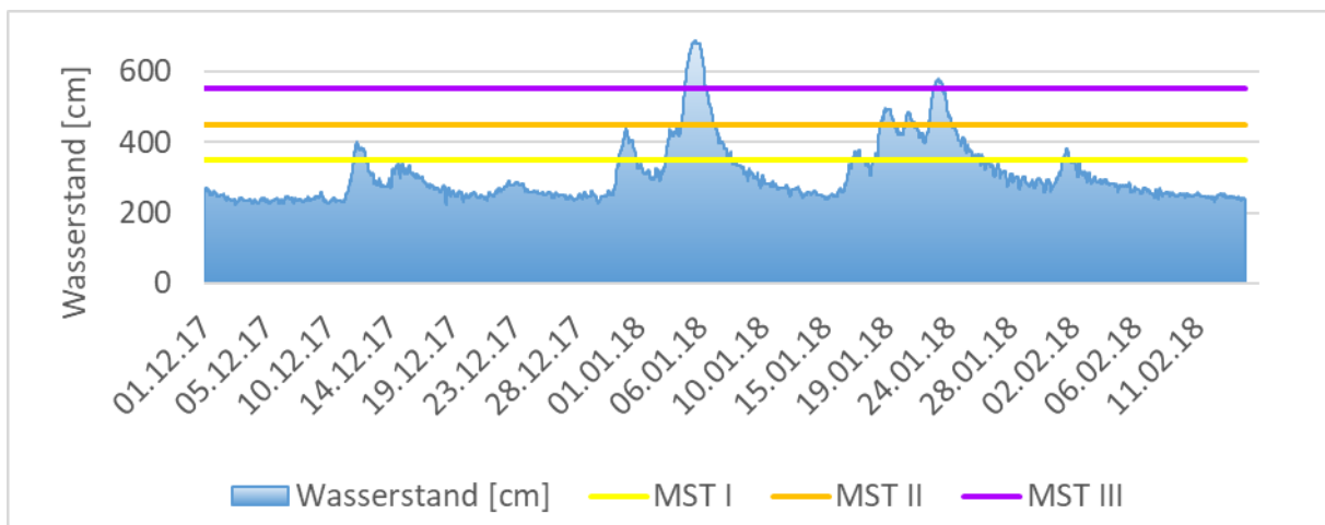
Abbildung 34: Wasserstand am Pegel Rockenau / Neckar. Meldestufe 1 = 350 cm (gelbe Linie), Meldestufe 2 = 450 cm (orangefarbene Linie), Meldestufe 3 = 550 cm (lila Linie)
