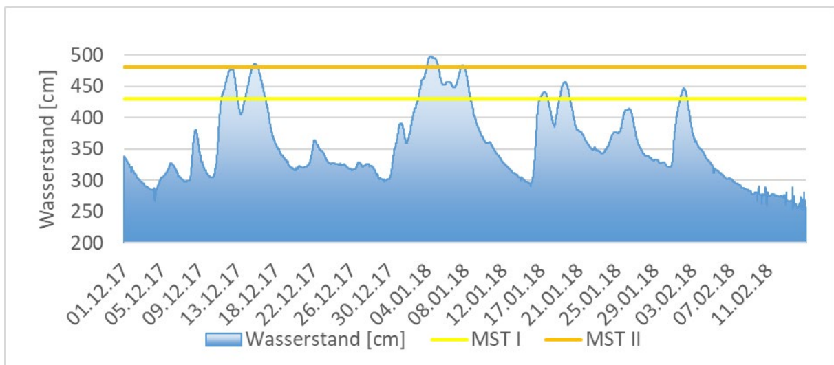
Abbildung 22: Wasserstand am Pegel Bad Hersfeld 1 / Fulda. Meldestufe 1 = 430 cm (gelbe Linie), Meldestufe 2 = 480 cm (orangefarbene Linie), Meldestufe 3 = 600 cm (nicht in Grafik zu sehen)
