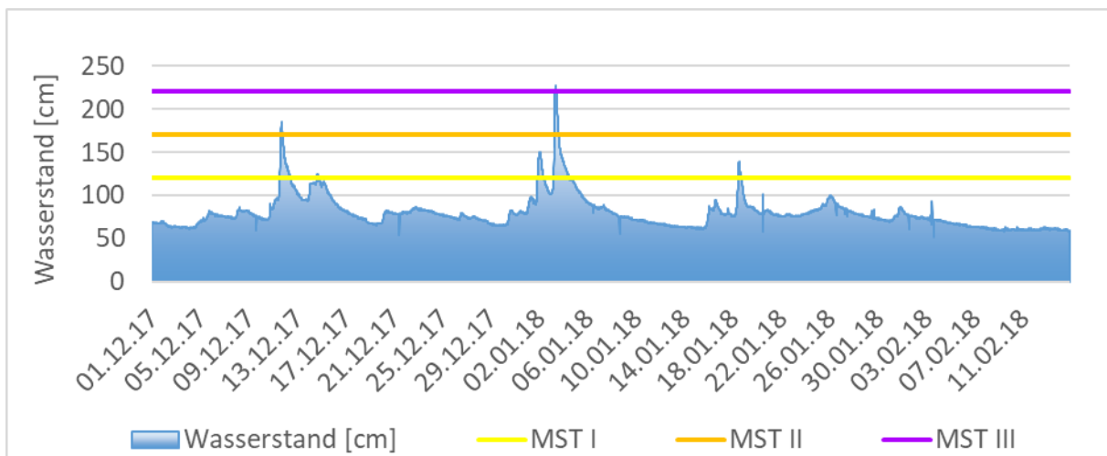
Abbildung 17: Wasserstand am Pegel Gemünden / Wohra. Meldestufe 1 = 120 cm (gelbe Linie), Meldestufe 2 = 170 cm (orangefarbene Linie), Meldestufe 3 = 220 cm (lila Linie)
