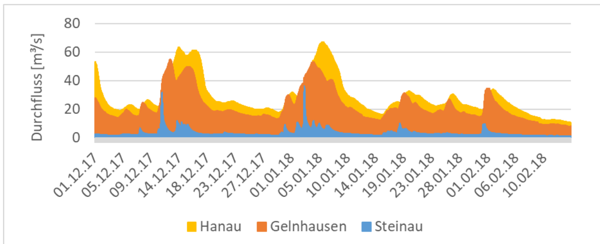
Abbildung 24: Durchflüsse der Kinzig
