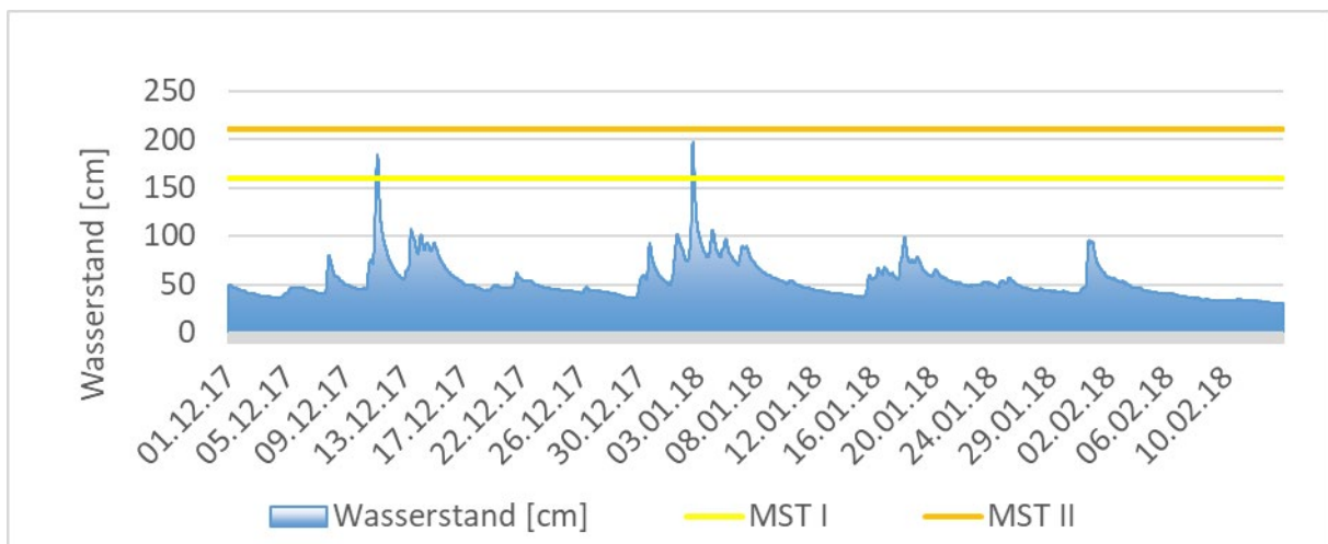
Abbildung 25: Wasserstand am Pegel Steinau / Kinzig. Meldestufe 1 = 160 cm (gelbe Linie), Meldestufe 2 = 210 cm (orangefarbene Linie), Meldestufe 3 = 270 cm (nicht in Grafik zu sehen)
