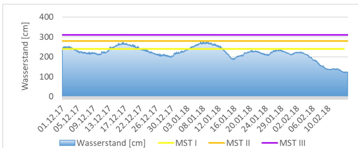
Abbildung 28: Wasserstand am Pegel Windecken / Nidder. Meldestufe 1 = 240 cm (gelbe Linie), Meldestufe 2 = 280 cm (orangefarbene Linie), Meldestufe 3 = 310 cm (lila Linie)
