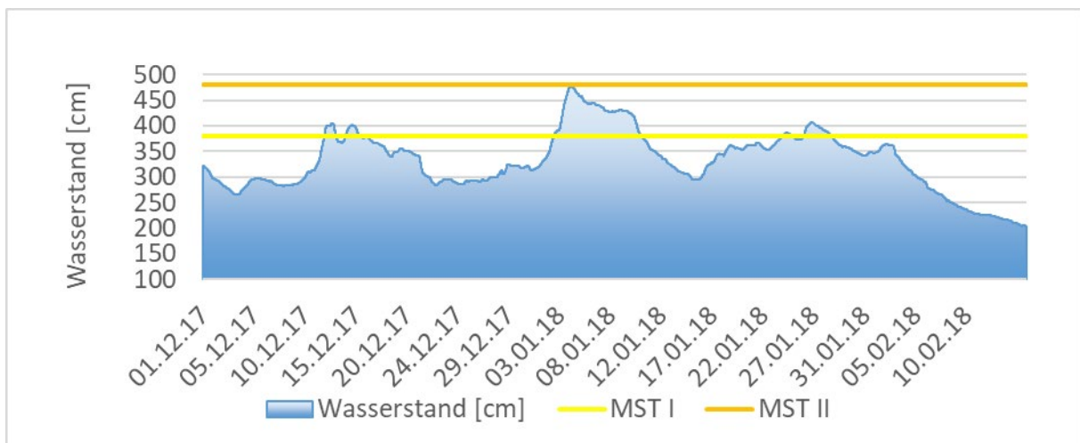
Abbildung 36: Wasserstand am Pegel Bad Karlshafen / Weser. Meldestufe 1 = 380 cm (gelbe Linie), Meldestufe 2 = 480 cm (orangefarbene Linie), Meldestufe 3 = 500 cm (nicht in Grafik zu sehen)
