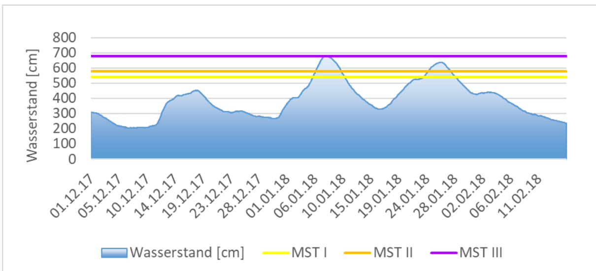
Abbildung 32: Wasserstand am Pegel Kaub / Rhein. Meldestufe 1 = 540 cm (gelbe Linie), Meldestufe 2 = 580 cm (orangefarbene Linie), Meldestufe 3 = 680 cm (lila Linie)
