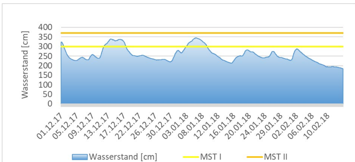
Abbildung 27: Wasserstand am Pegel Hanau / Kinzig. Meldestufe 1 = 300 cm (gelbe Linie), Meldestufe 2 = 370 cm (orangefarbene Linie), Meldestufe 3 = 440 cm (nicht in Grafik zu sehen)
