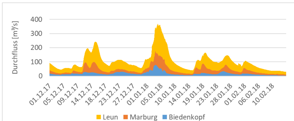
Abbildung 12: Durchflüsse an der Lahn
