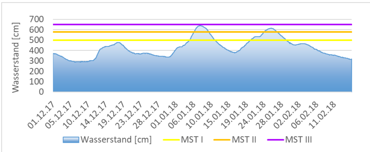
Abbildung 31: Wasserstand am Pegel Mainz / Rhein. Meldestufe 1 = 500 cm (gelbe Linie), Meldestufe 2 = 580 cm (orangefarbene Linie), Meldestufe 3 = 650 cm (lila Linie)
