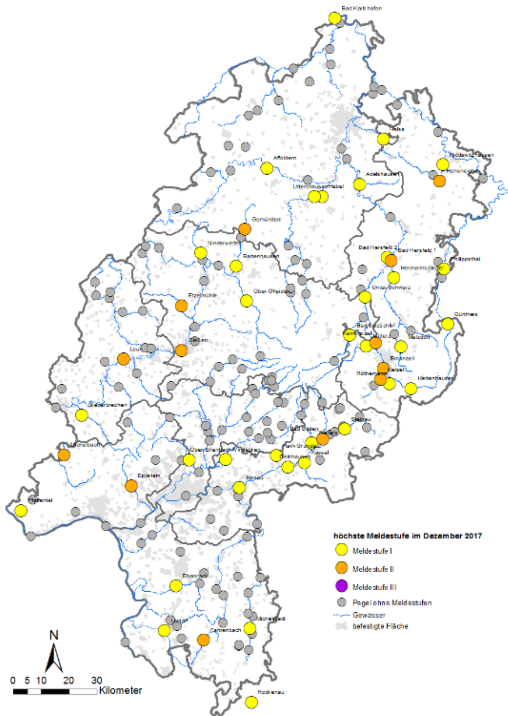
Abbildung 9: Meldestufenüberschreitungen Dezember 2017
