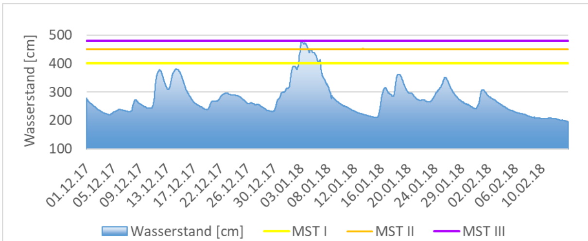
Abbildung 14: Wasserstand am Pegel Marburg / Lahn. Meldestufe 1 = 400 cm (gelbe Linie), Meldestufe 2 = 450 cm (orangefarbene Linie), Meldestufe 3 = 480 cm (lila Linie)
