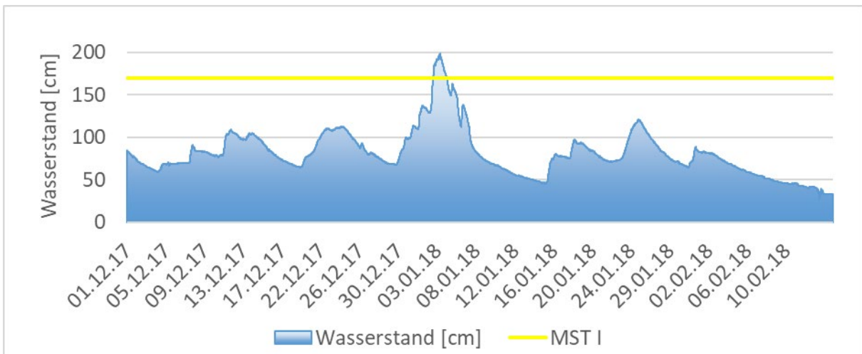
Abbildung 13: Wasserstand am Pegel Biedenkopf / Lahn. Meldestufe 1 = 170 cm (gelbe Linie), Meldestufe 2 = 210 cm (nicht in Grafik zu sehen), Meldestufe 3 = 270 cm (nicht in Grafik zu sehen)
