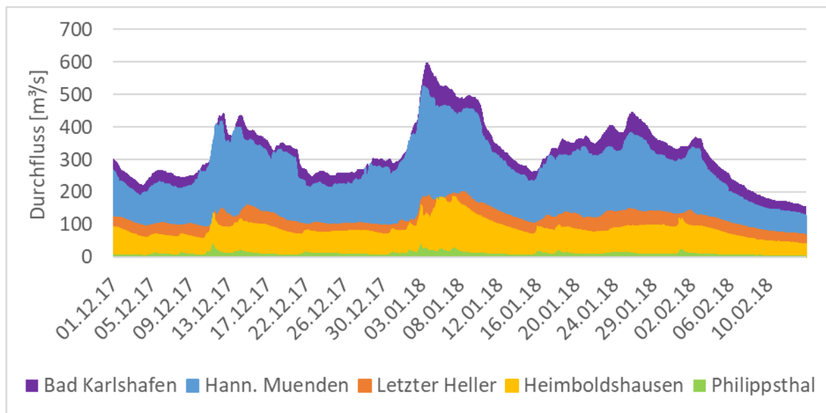
Abbildung 35: Durchflüsse in Weser, Werra und Ulster
