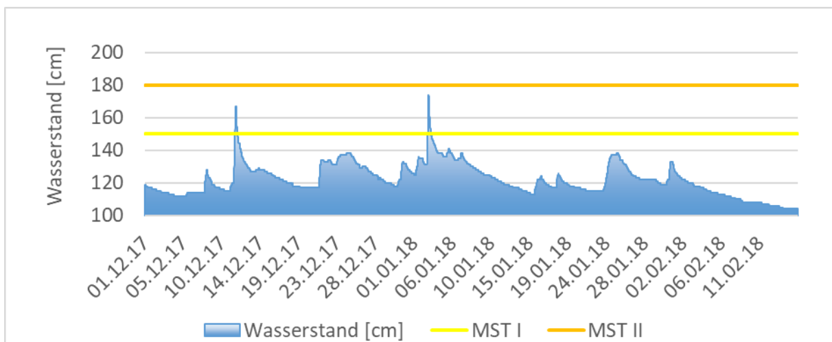
Abbildung 20: Wasserstand am Pegel Hettenhausen / Fulda. Meldestufe 1 = 150 cm (gelbe Linie), Meldestufe 2 = 180 cm (orangefarbene Linie), Meldestufe 3 = 210 cm (nicht in Grafik zu sehen)
