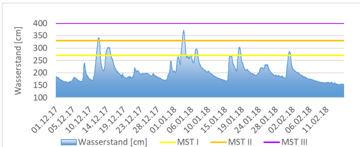
Abbildung 21: Wasserstand am Pegel Kämmerzell / Fulda. Meldestufe 1 = 270 cm (gelbe Linie), Meldestufe 2 = 330 cm (orangefarbene Linie), Meldestufe 3 = 400 cm (lila Linie)
