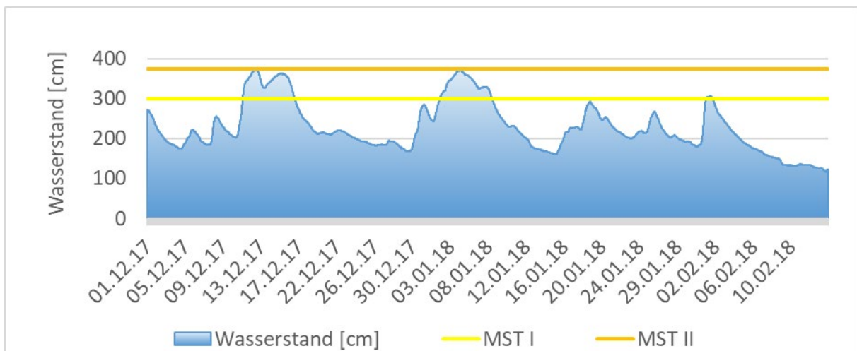
Abbildung 26: Wasserstand am Pegel Gelnhausen / Kinzig. Meldestufe 1 = 300 cm (gelbe Linie), Meldestufe 2 = 375 cm (orangefarbene Linie), Meldestufe 3 = 460 cm (nicht in Grafik zu sehen)
