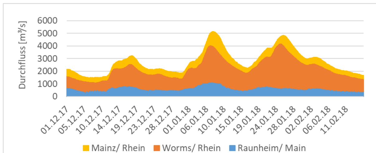
Abbildung 29: Durchflüsse in Rhein und Main
