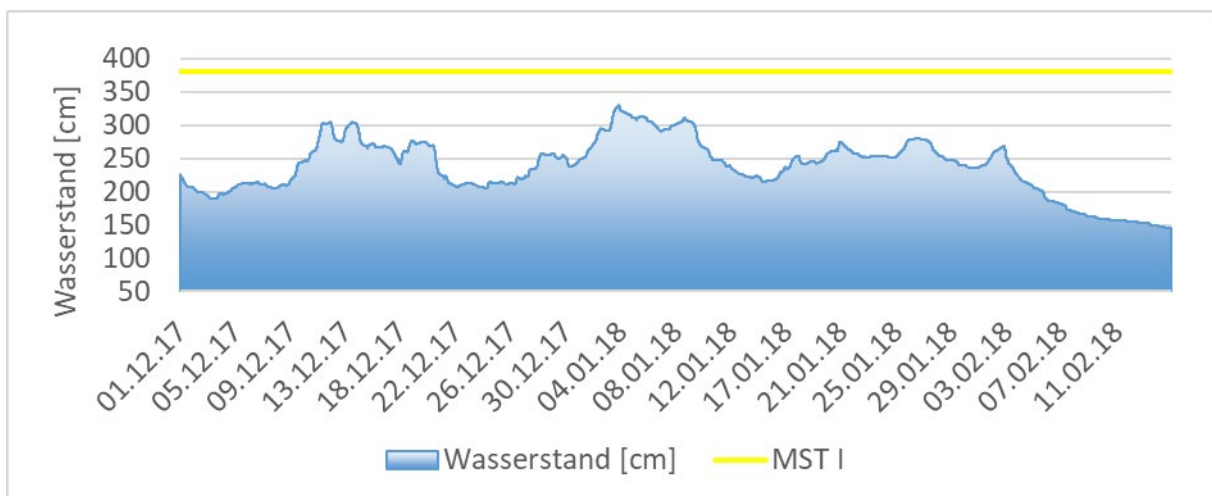
Abbildung 23: Wasserstand am Pegel Gunterhausen / Fulda. Meldestufe 1 = 380 cm (gelbe Linie), Meldestufe 2 = 410 cm (nicht in Grafik zu sehen), Meldestufe 3 = 450 cm (nicht in Grafik zu sehen)
