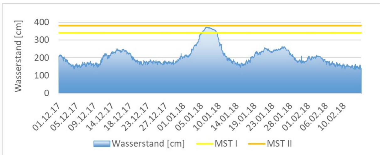
Abbildung 33: Wasserstand am Pegel Raunheim / Main. Meldestufe 1 = 340 cm (gelbe Linie), Meldestufe 2 = 380 cm (orangefarbene Linie), Meldestufe 3 = 470 cm (nicht in Grafik zu sehen)
