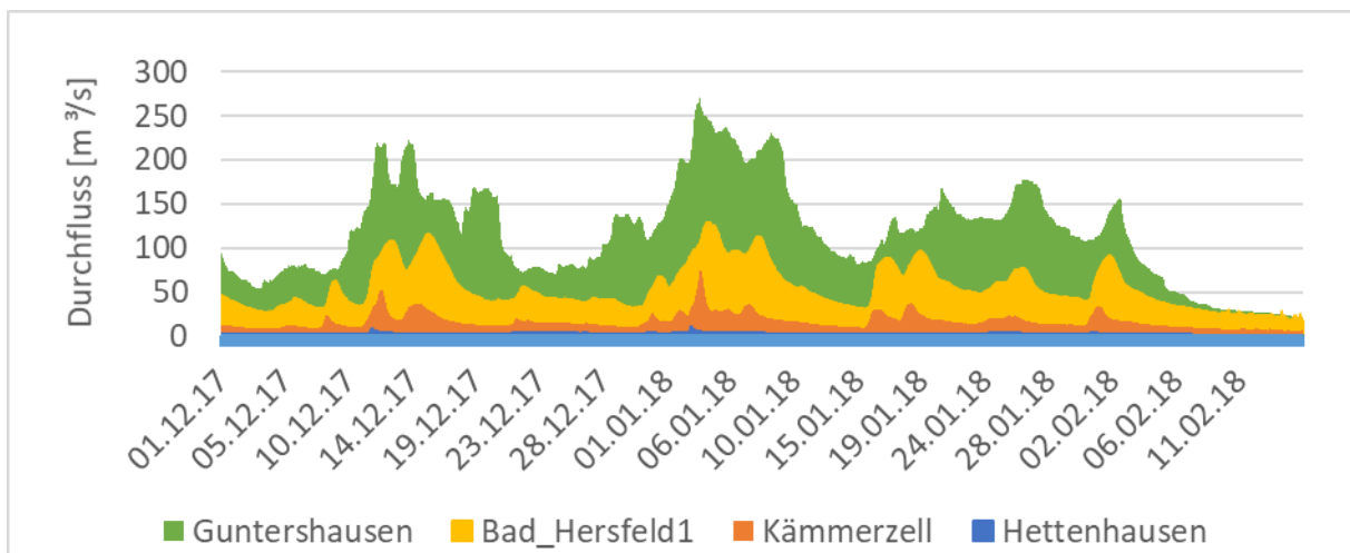
Abbildung 19: Durchflüsse der Fulda
