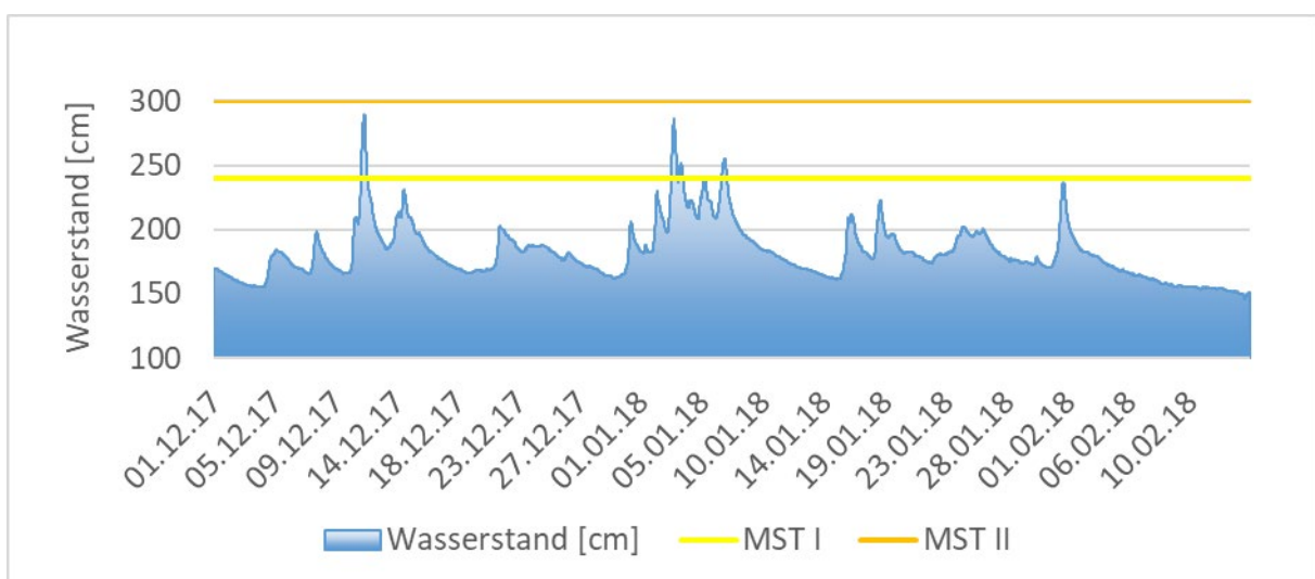
Abbildung 38: Wasserstand am Pegel Philippsthal / Ulster. Meldestufe 1 = 240 cm (gelbe Linie), Meldestufe 2 = 300 cm (orangefarbene Linie), Meldestufe 3 = 340 cm (nicht in Grafik zu sehen)
