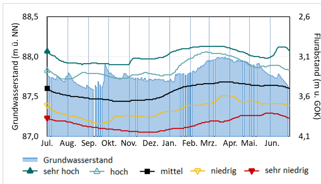
Abbildung 19: Grundwasserganglinie der Messstelle Bürstadt
