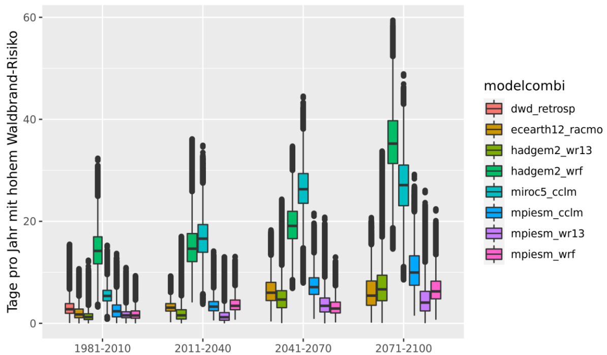
Abb. 2: Mittlere Anzahl der Tage im Jahr mit einem hohen Waldbrandrisiko für die Waldflächen in Hessen
