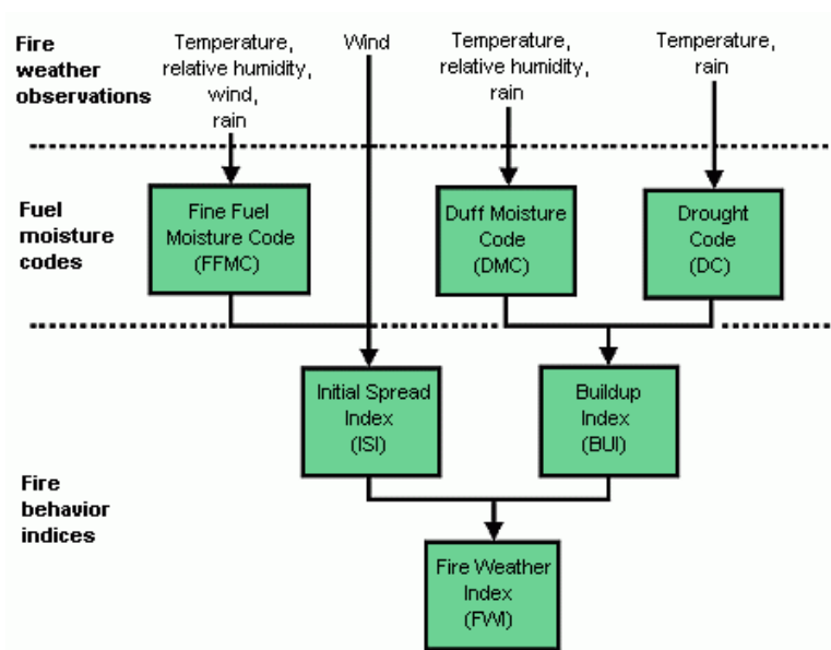
Abb. 1: Komponenten des FWI Index (Natural Resources Canada, 2008)
