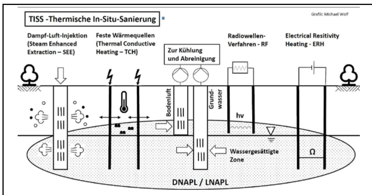
Abb. 1: Thermische In-Situ-Sanierung – Verfahren (Kap. 2.1–2.4) © Michael Wolf
