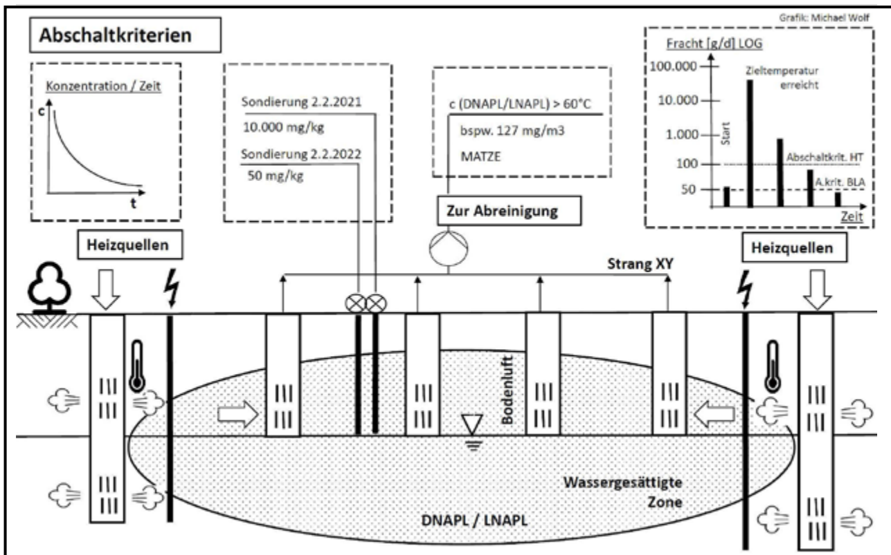
Abb. 2: Abschaltkriterien für TISS (Kap. 4.1-4.4) © Michael Wolf
