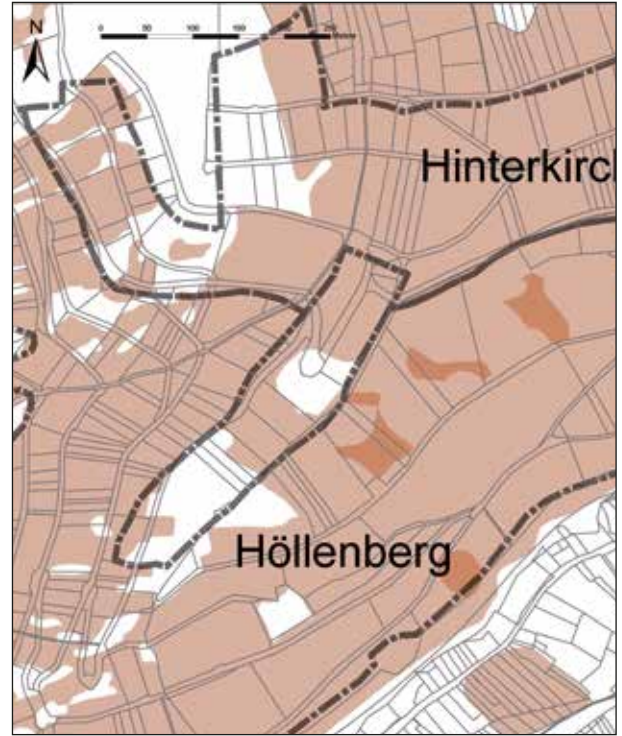
Abb. 30: Lage mit homogenen Substraten – Hinterkirch/Höllenberg (Mittelrhein) (Legende siehe Abb. 28).
