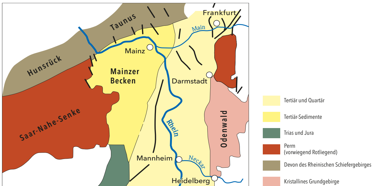
Abb. 5: Geologische Übersichtskarte der hessischen Weinbaugebiete.
