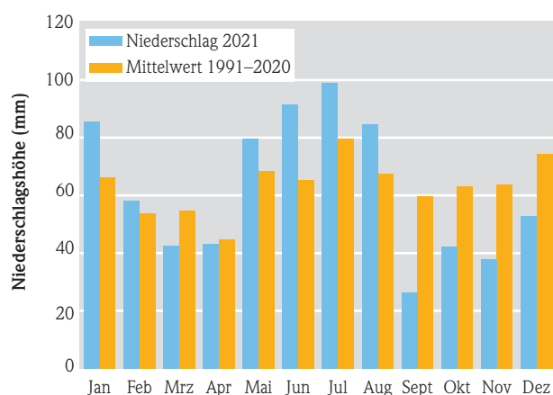
Abb. 2: Niederschlagshöhe in Hessen, Datenquelle: Deutscher Wetterdienst
