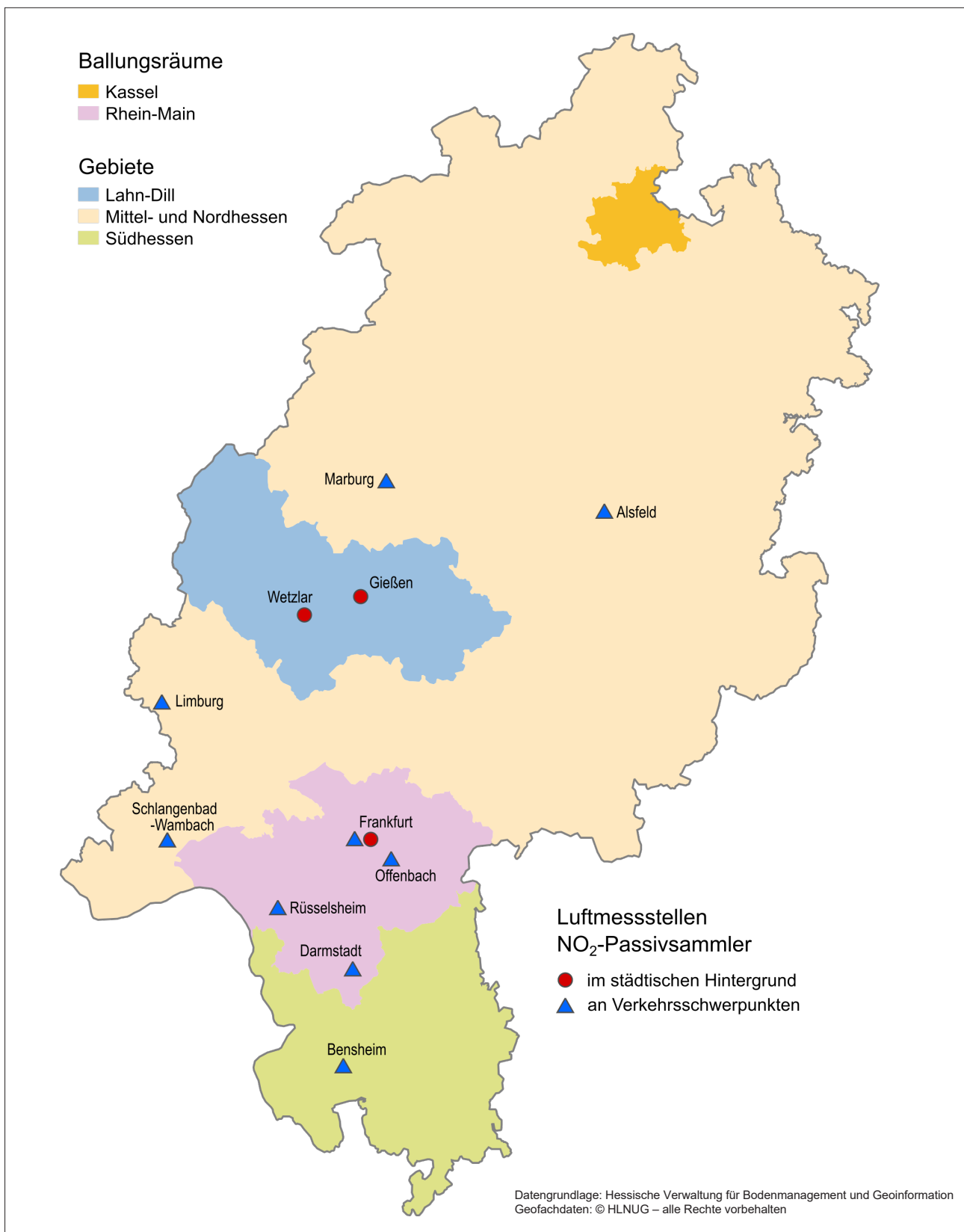
Abb. 19: Luftmessstellen mit NO 2 -Passivsammllern (Stand 2021). In einzelnen Städten werden mehrere Passivsammllern eingesetzt, Details sind der Tabelle zur Geräteausstattung der Luftmessstellen zu entnehmen.
