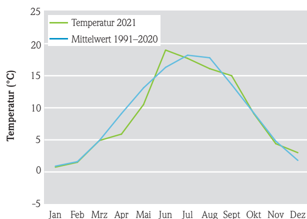
Abb. 1: Temperatur in Hessen, Datenquelle: Deutscher Wetterdienst
