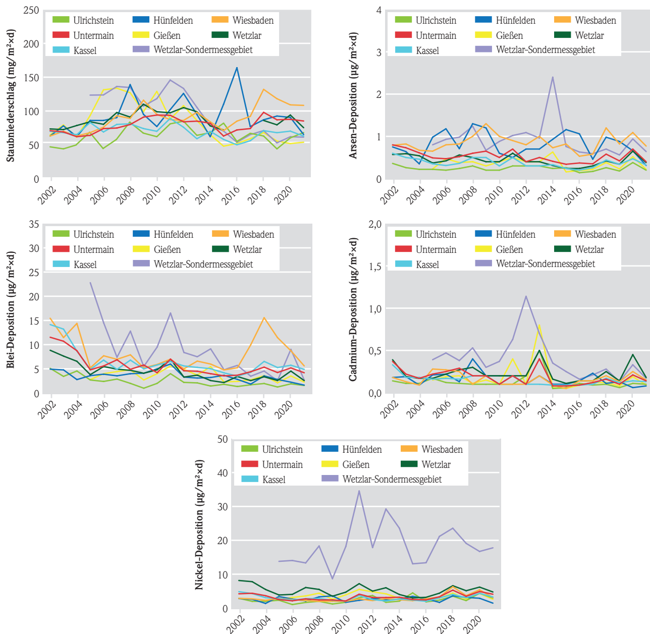
Abb. 16: Zeitreihen der mittleren Belastung durch Staubbiederschlag und dessen Inhaltsstoffe 2002–2021
