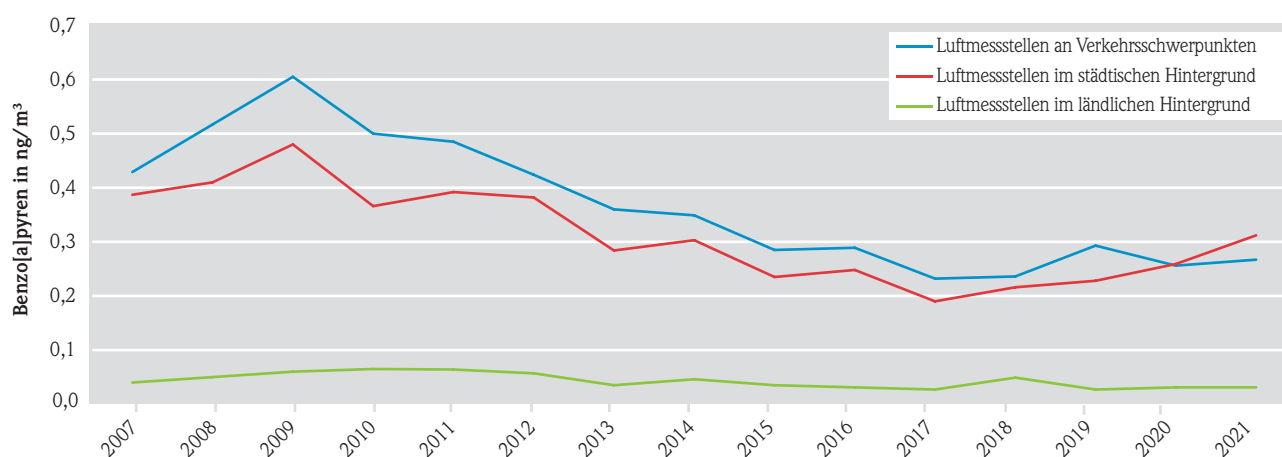
Abb. 15: Zeitreihe der Jahresmittelwerte 2007–2021, Benzo[a]pyren als Bestandteil des Feinstaubs PM 10 . Für die Ermittlung der Jahresmittelwerte wurde ein arithmetisches Mittel über alle Messstellen gleichen Charakters (Verkehrsschwerpunkte, städtischer Hintergrund, ländlicher Hintergrund) in ganz Hessen gebildet. Dabei wurden die Werte aller im jeweiligen Jahr verfügbaren Messstellen zur Berechnung herangezogen.
