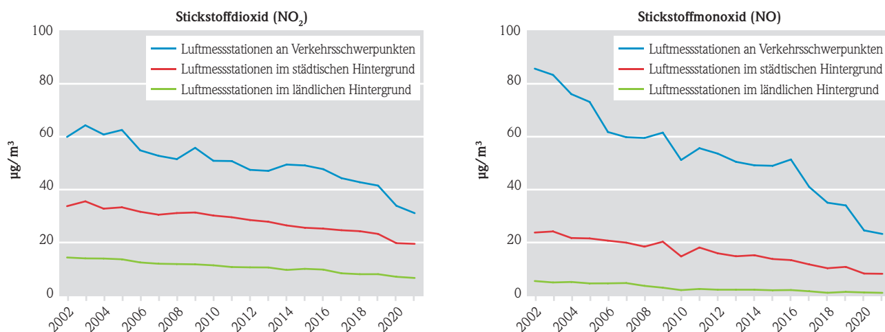
Abb. 5: Zeitreihen der Jahresmittelwerte 2002–2021 an Messstellen für Stickstoffdioxid und Stickstoffmonoxid. Für die Ermittlung der Jahresmittelwerte wurde ein arithmetisches Mittel über alle Luftmessstellen gleichen Charakters (Verkehrsschwerpunkte, städtischer Hintergrund, ländlicher Hintergrund) in ganz Hessen gebildet. Dabei wurden die Werte aller im jeweiligen Jahr verfügbaren Messstellen, die zur Beurteilung der Luftqualität herangezogen werden, in der Berechnung verwendet.
