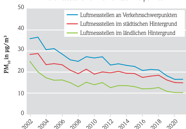
Abb. 12: Zeitreihen der Jahresmittelwerte 2002–2021, Feinstaub PM 10 und Feinstaub PM 2,5 . Für die Ermittlung der Jahresmittelwerte wurde ein arithmetisches Mittel über alle Messstellen gleichen Charakters (Verkehrsschwerpunkte, städtischer Hintergrund, ländlicher Hintergrund) in ganz Hessen gebildet. Dabei wurden die Werte aller im jeweiligen Jahr verfügbaren Messstellen zur Berechnung herangezogen.
